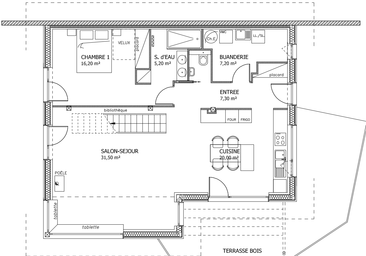
PLAN REZ DE CHAUSSÉE
