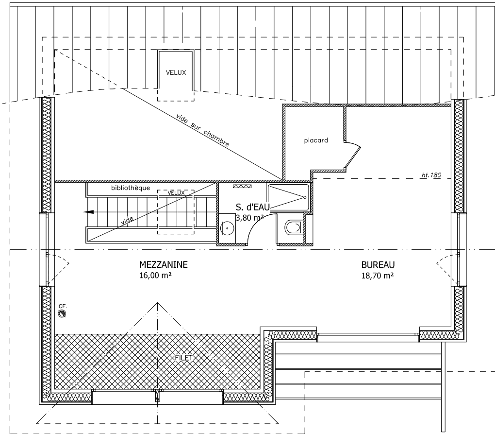
PLAN ÉTAGE
