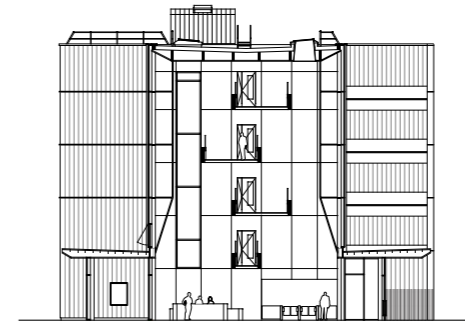
Coupe AA' Ech: 1:500
