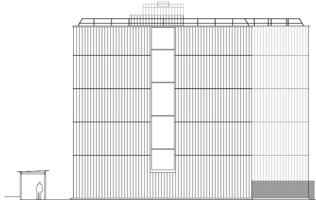
Élévation sud Ech: 1:250
