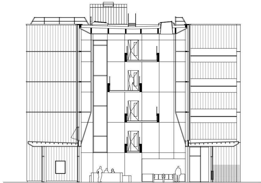
Coupe AA' Ech: 1:250
