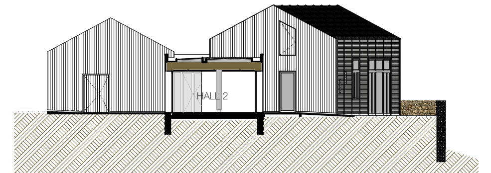
COUPE TRANSVERSALE CT.3
