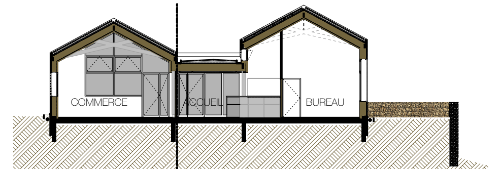
COUPE TRANSVERSALE CT.2
