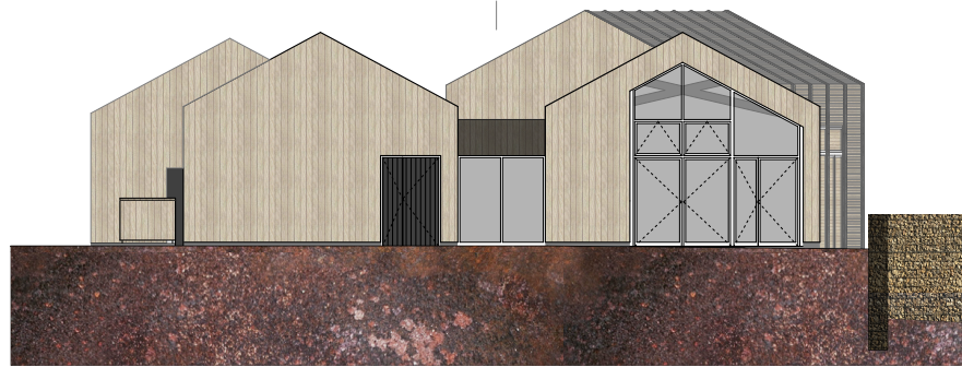
ELÉVATION EST - CÔTÉ TERRASSE RESTAURANT
