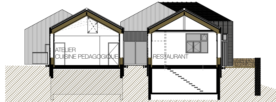
COUPE TRANSVERSALE CT.4
