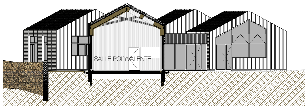
COUPE TRANSVERSALE CT.1
