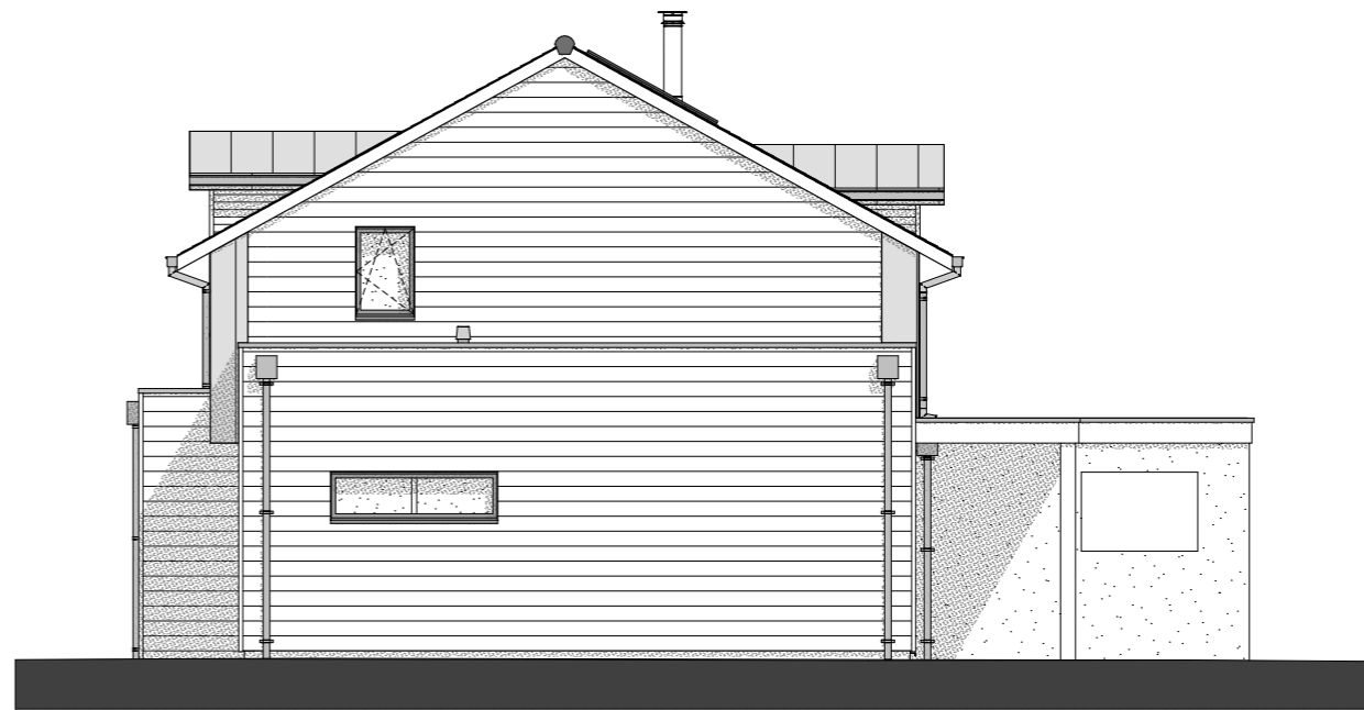
FAÇADE OUEST
