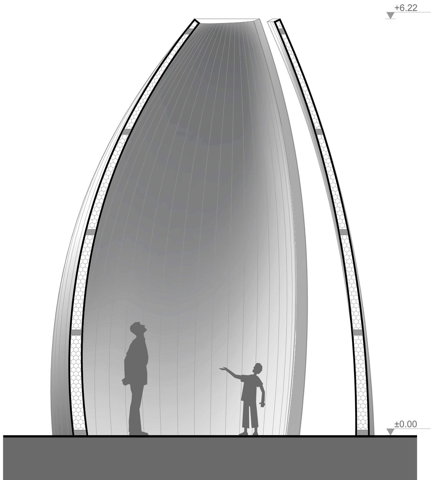
Coupe
