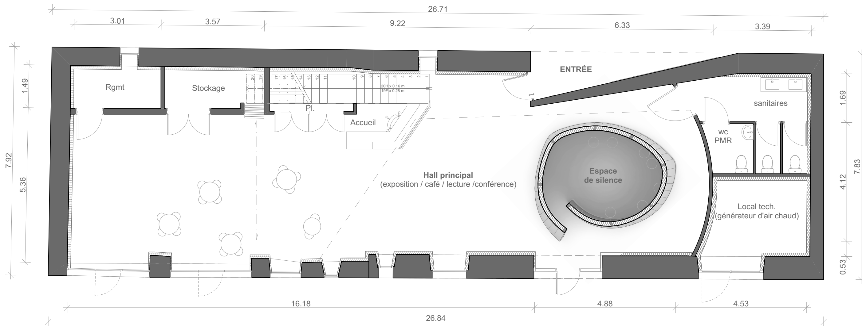
Plan RDC
