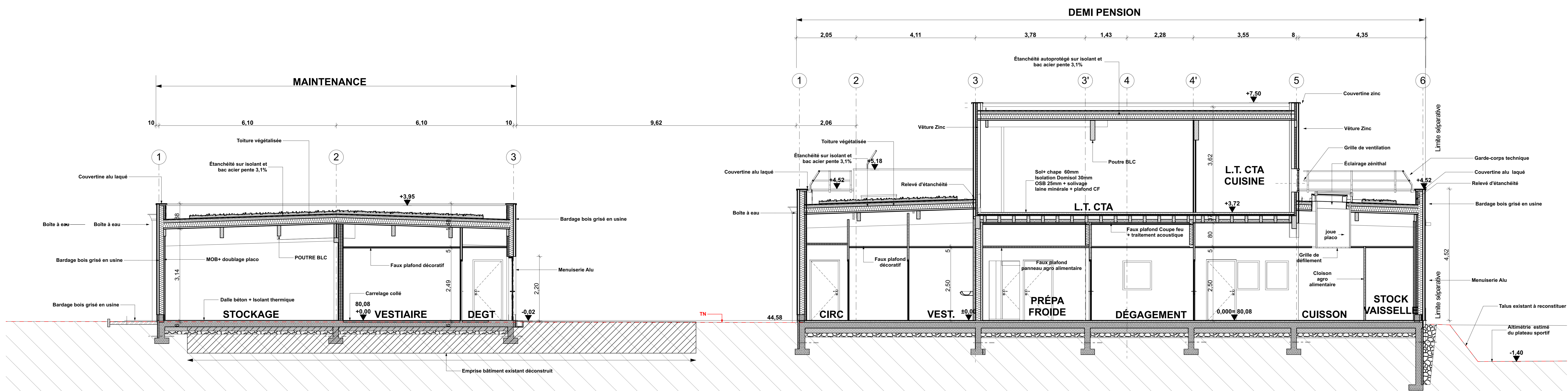
COUPE C - C
