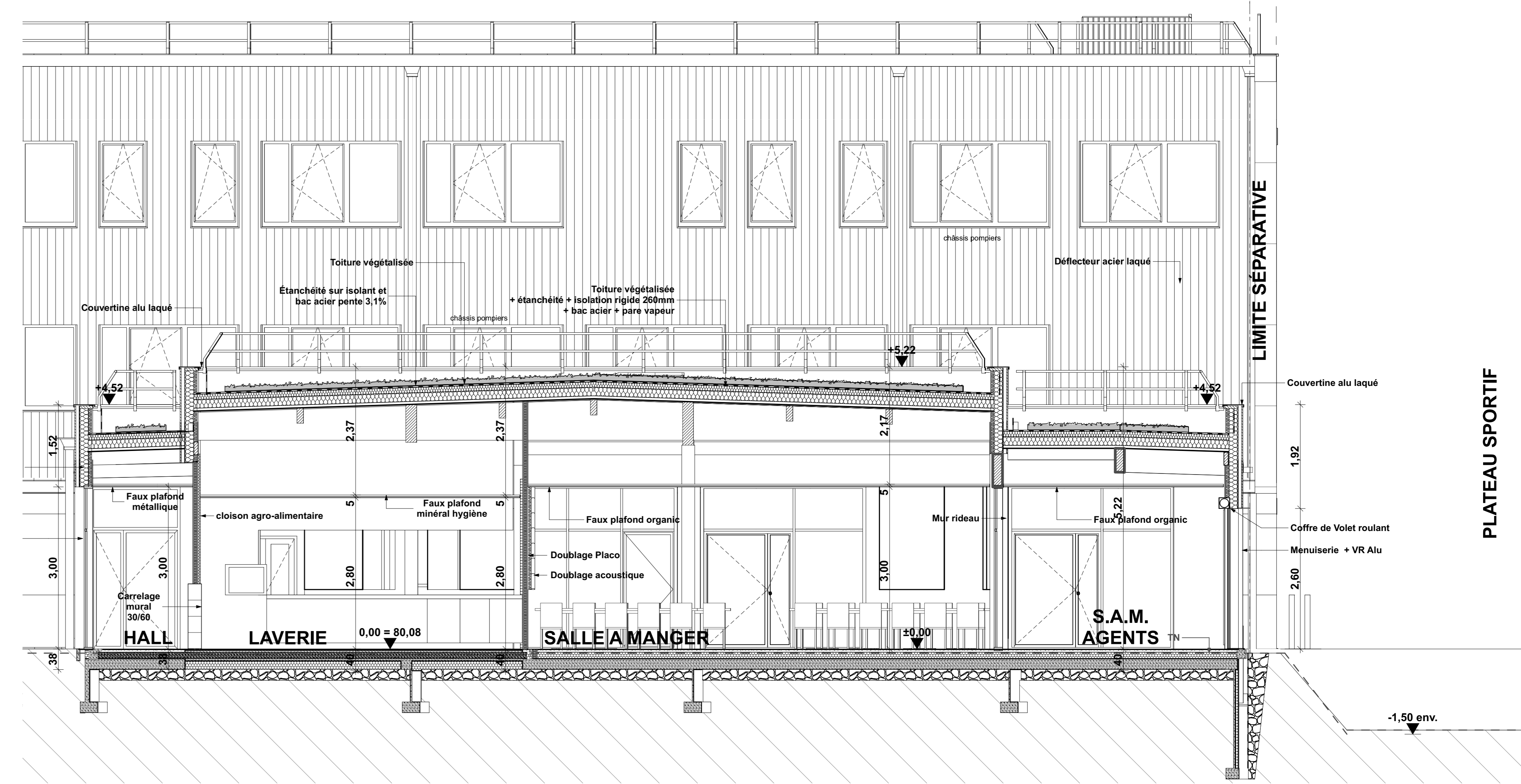
COUPE B - B
