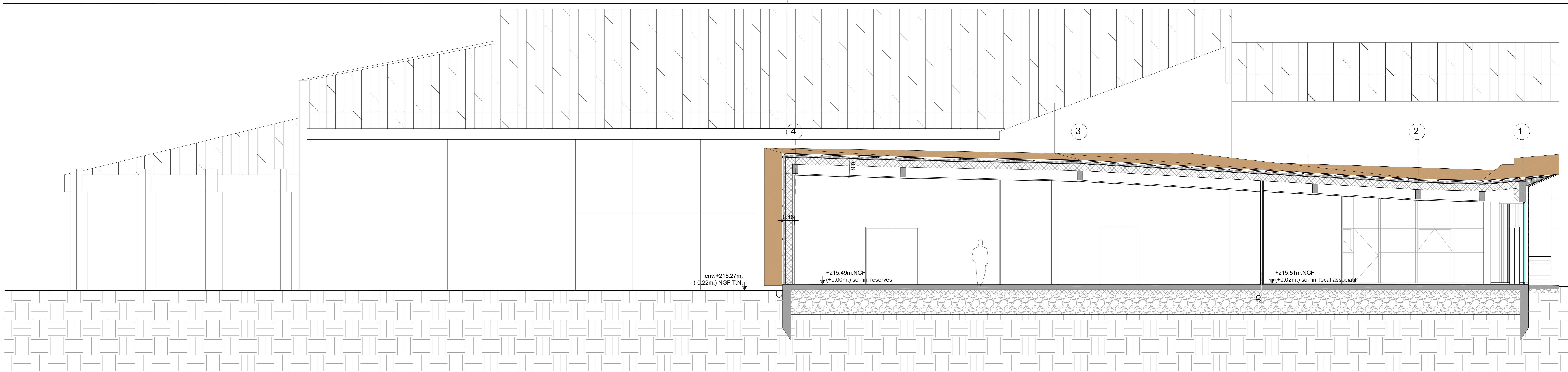
01 Coupe AA 1:50
