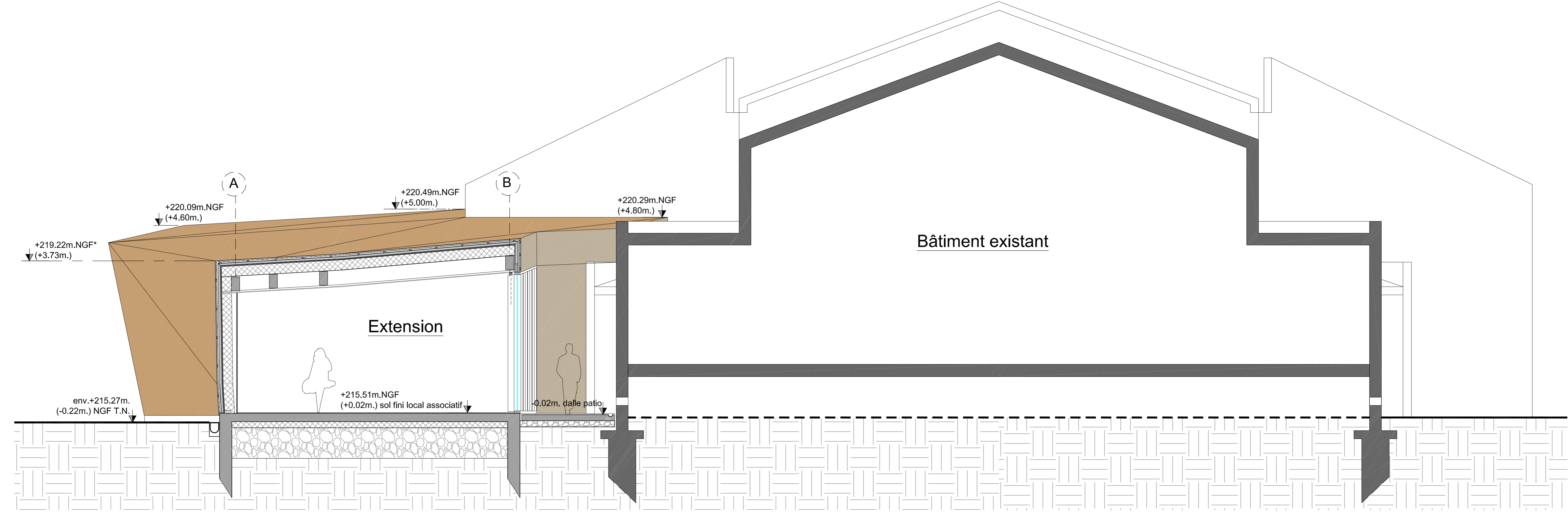
02 Coupe BB 1:50
