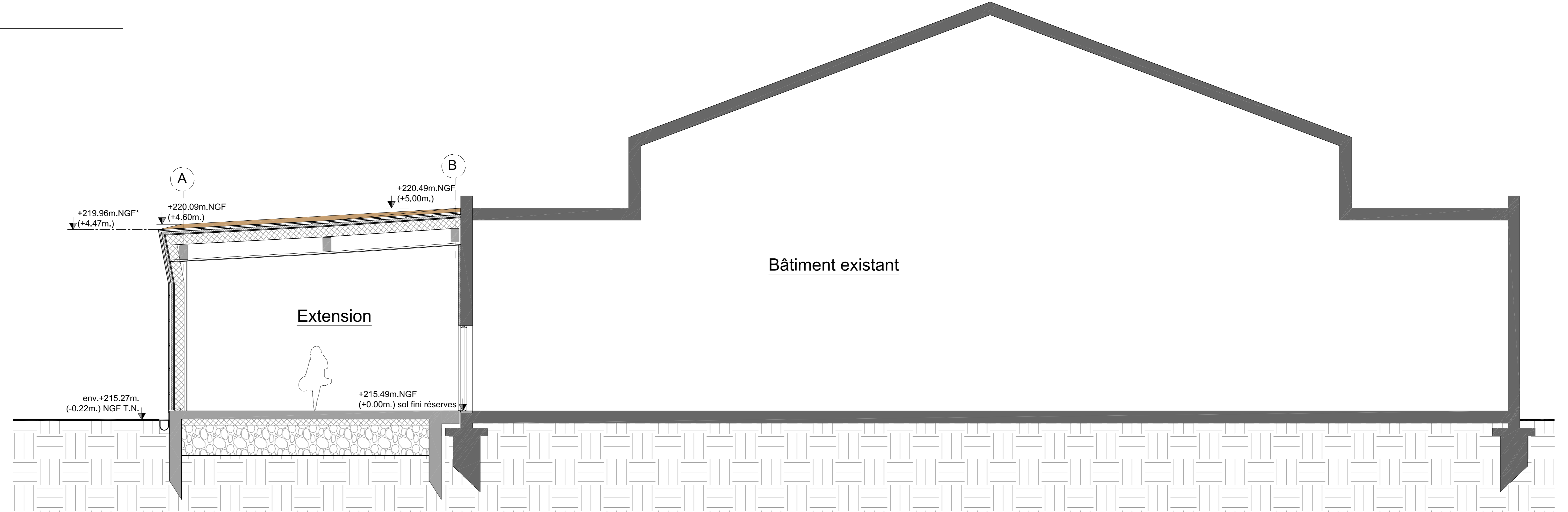
03 Coupe CC 1:50
