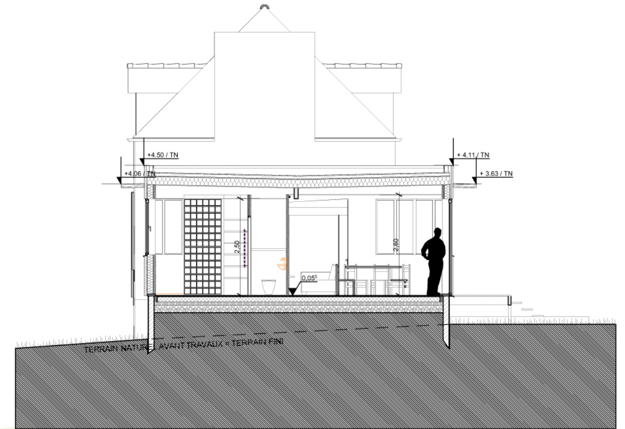
Coupe BB
