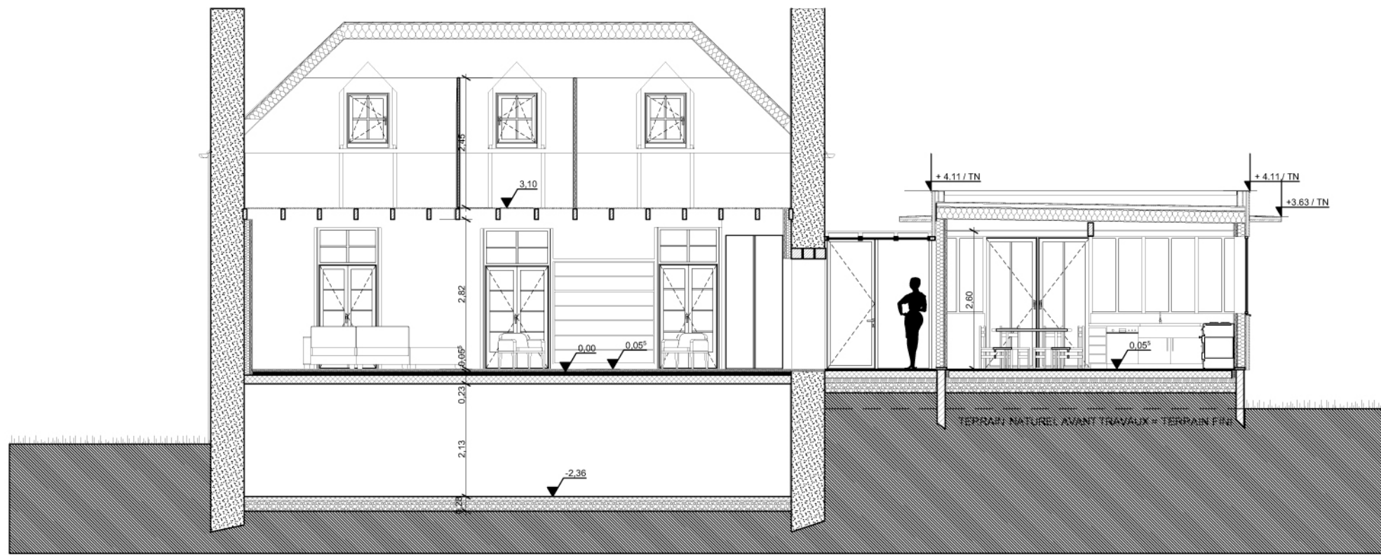
Coupe AA
