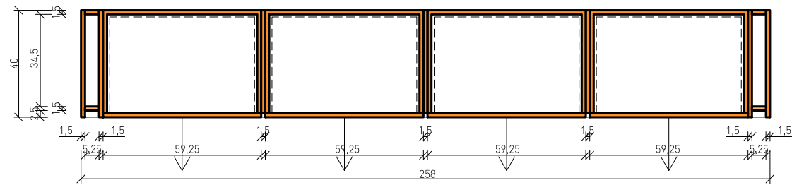
Alignement sur dessus le bas du rampant
