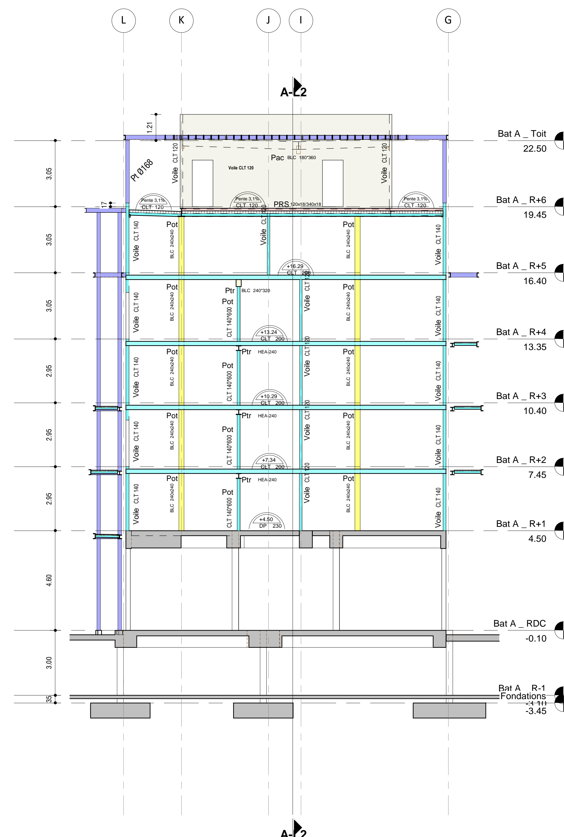
COUPE T2
