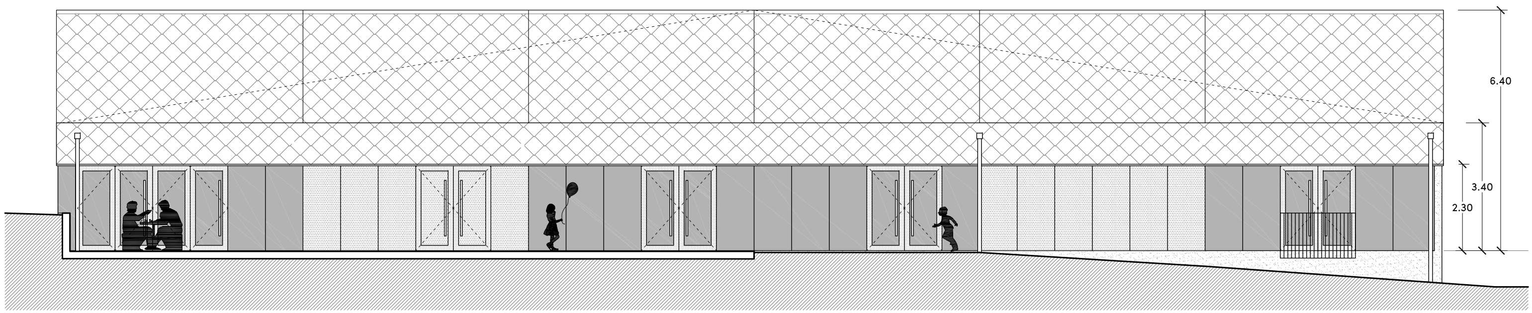
façade ouest
