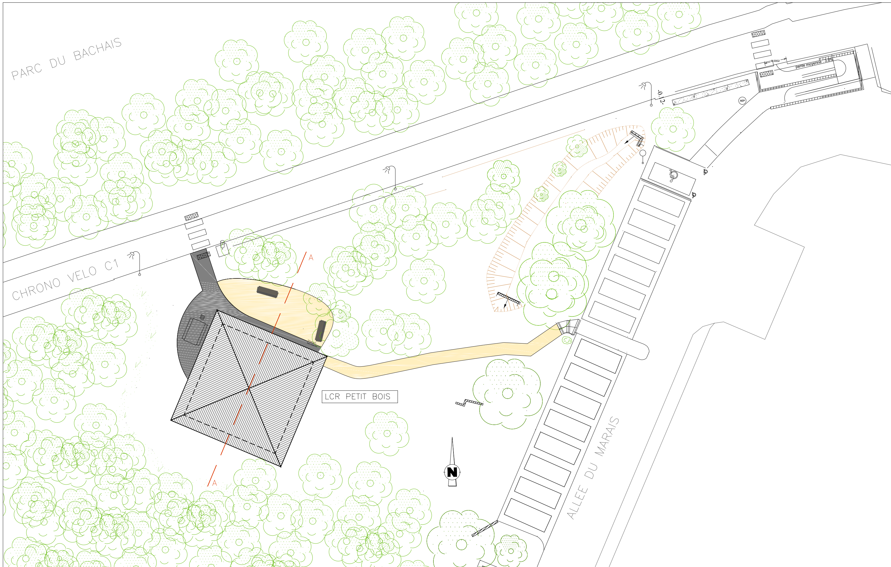
LCR PETIT BOIS PLAN DE MASSE ECH 1/200 SERVICE CONSTRUCTION DURABLE _ VILLE DE MEYLAN
