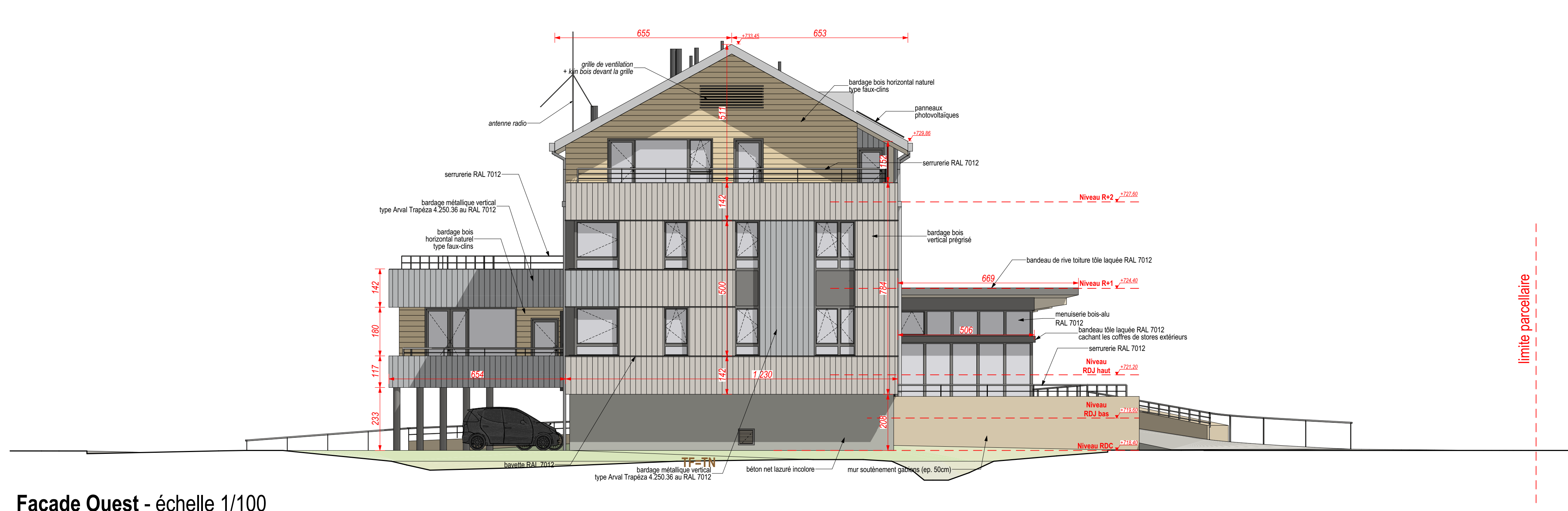
Façade Ouest - échelle 1/100
