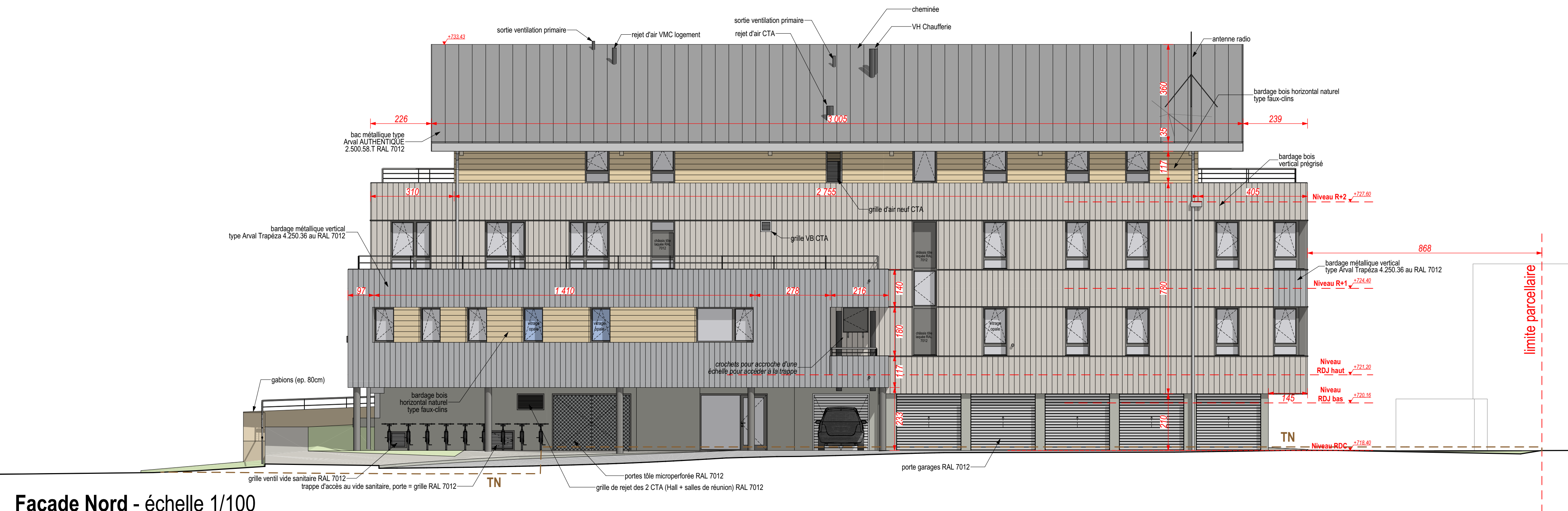
Façade Nord - échelle 1/100
