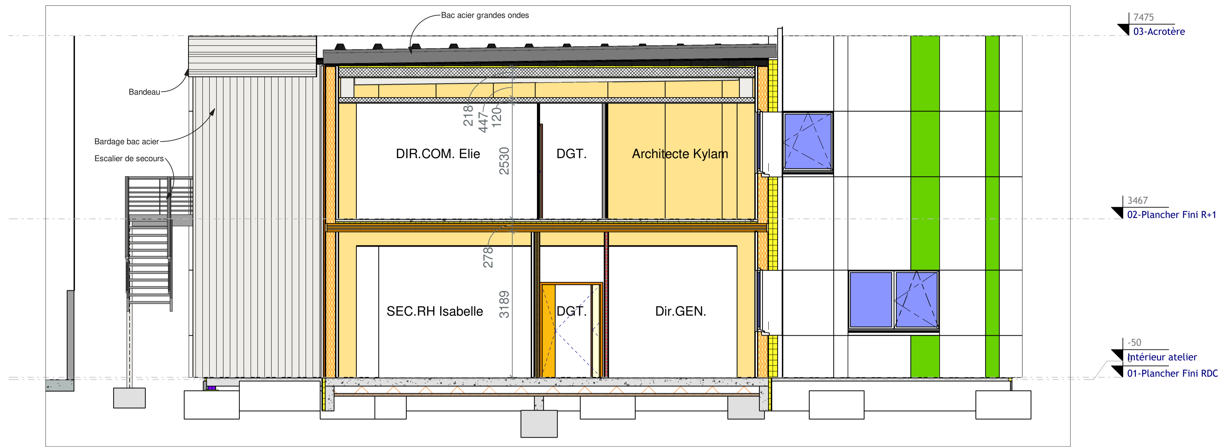
2 Coupe 2 Ech : 1 : 50
