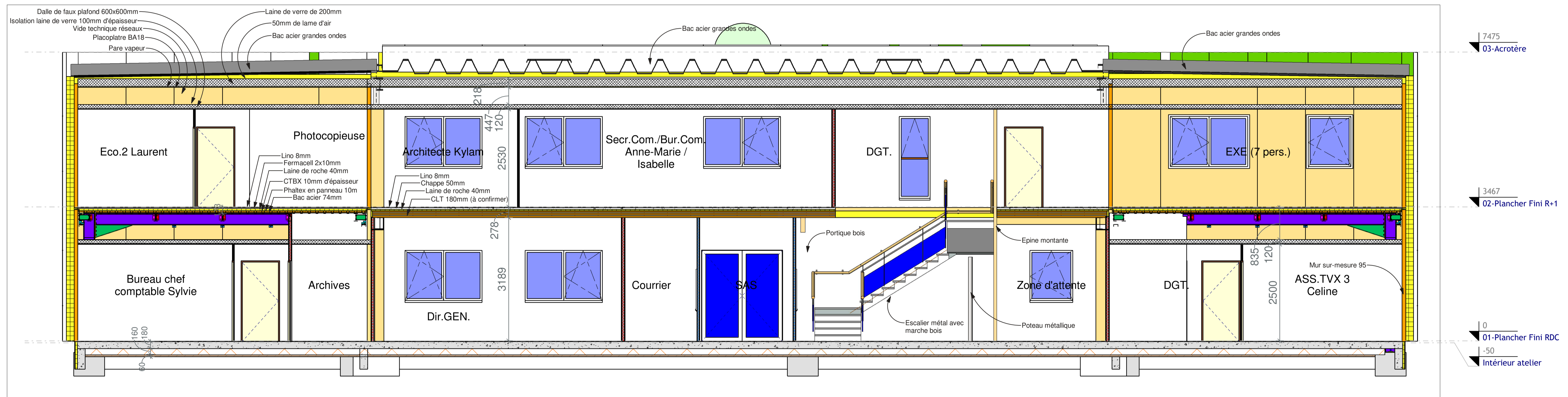
3 Coupe 3 Ech : 1 : 50
