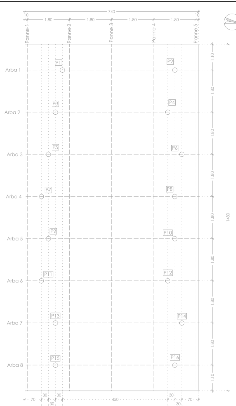
PLAN DE TOITURE - 1/50
