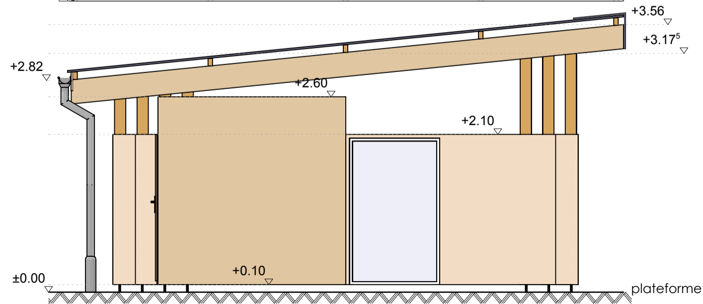
COUPE TRANSVERSALE - 1/50
