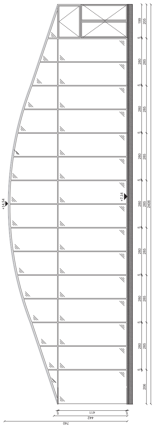
ELEVATION PRINCIPALE
