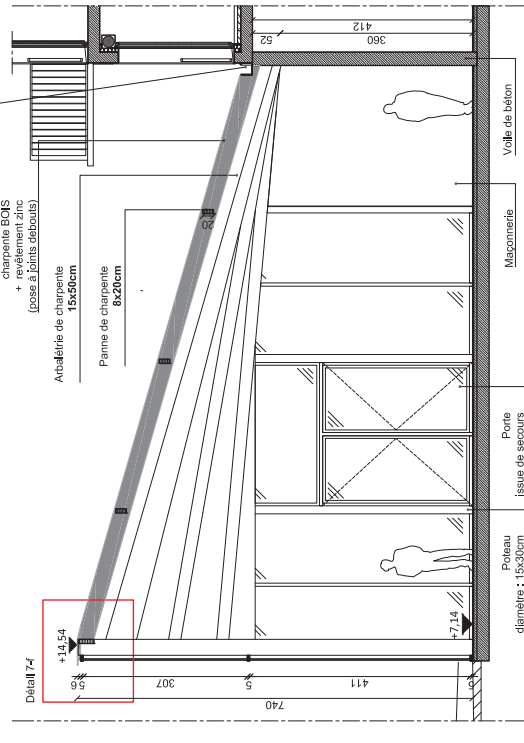
COUPE TRANSVERSALE
