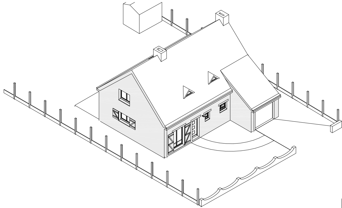
ETAT EXISTANT Axonométries sud & ouest
