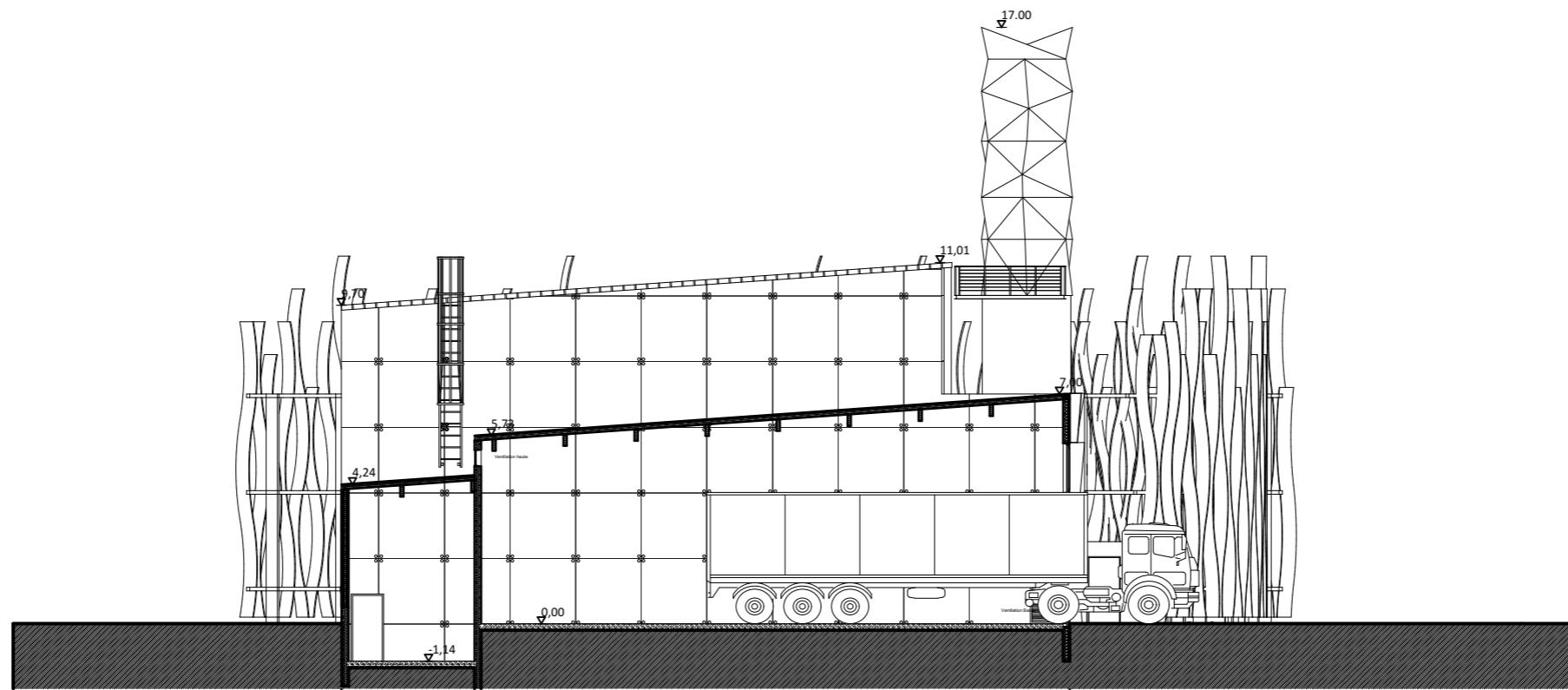
Coupe CC
