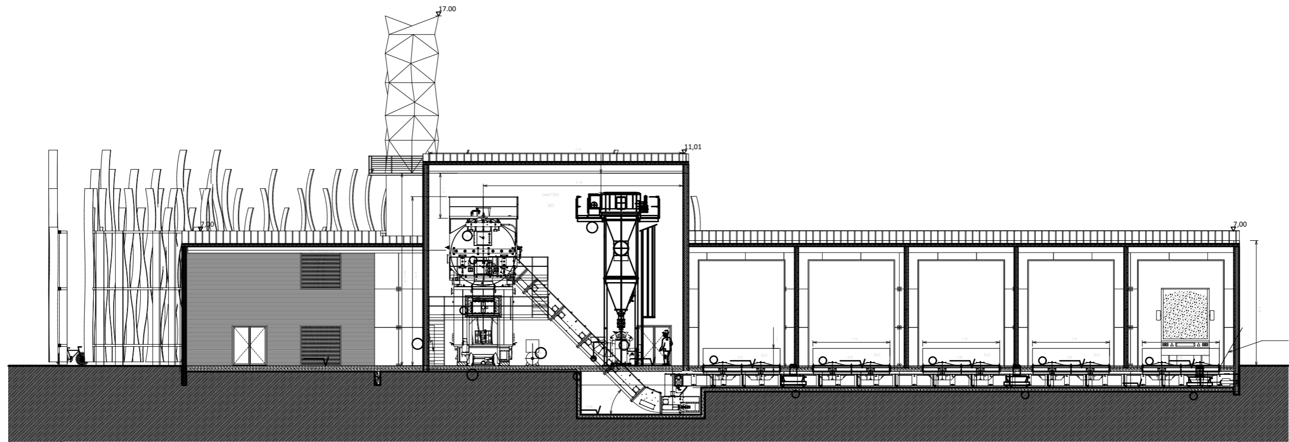
Coupe AA
