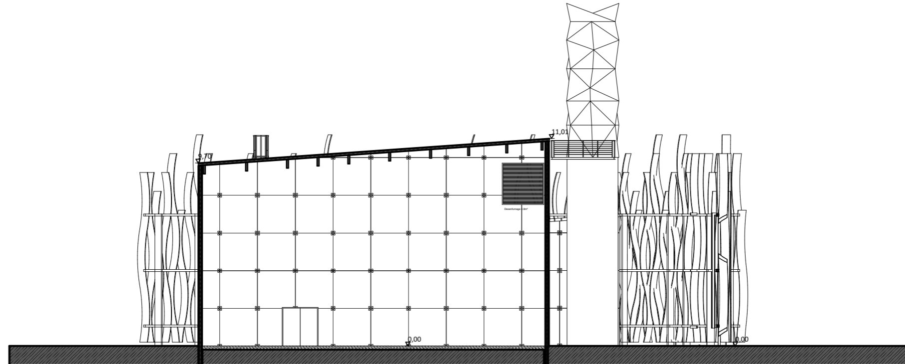
Coupe BB
