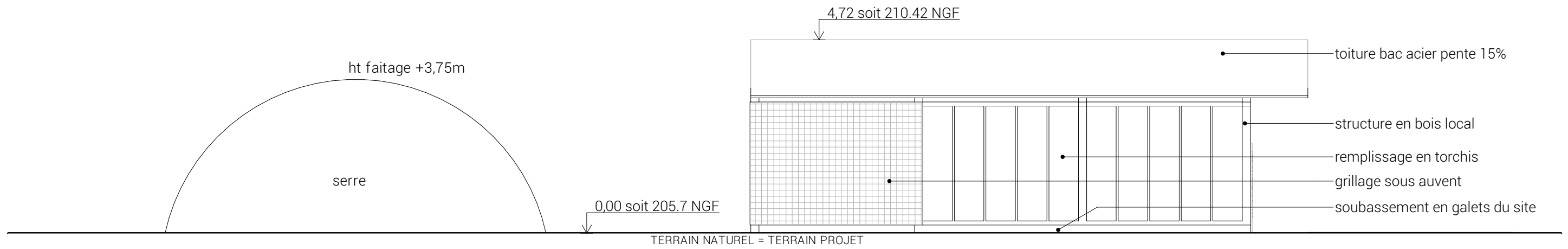
Façade Sud
