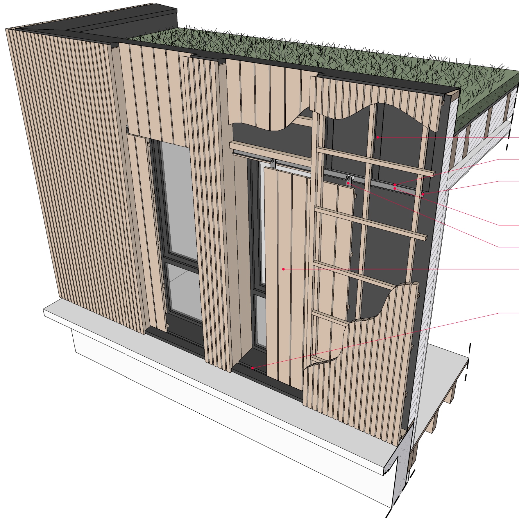
Détail Volets Coulissants Menuiseries R+1
