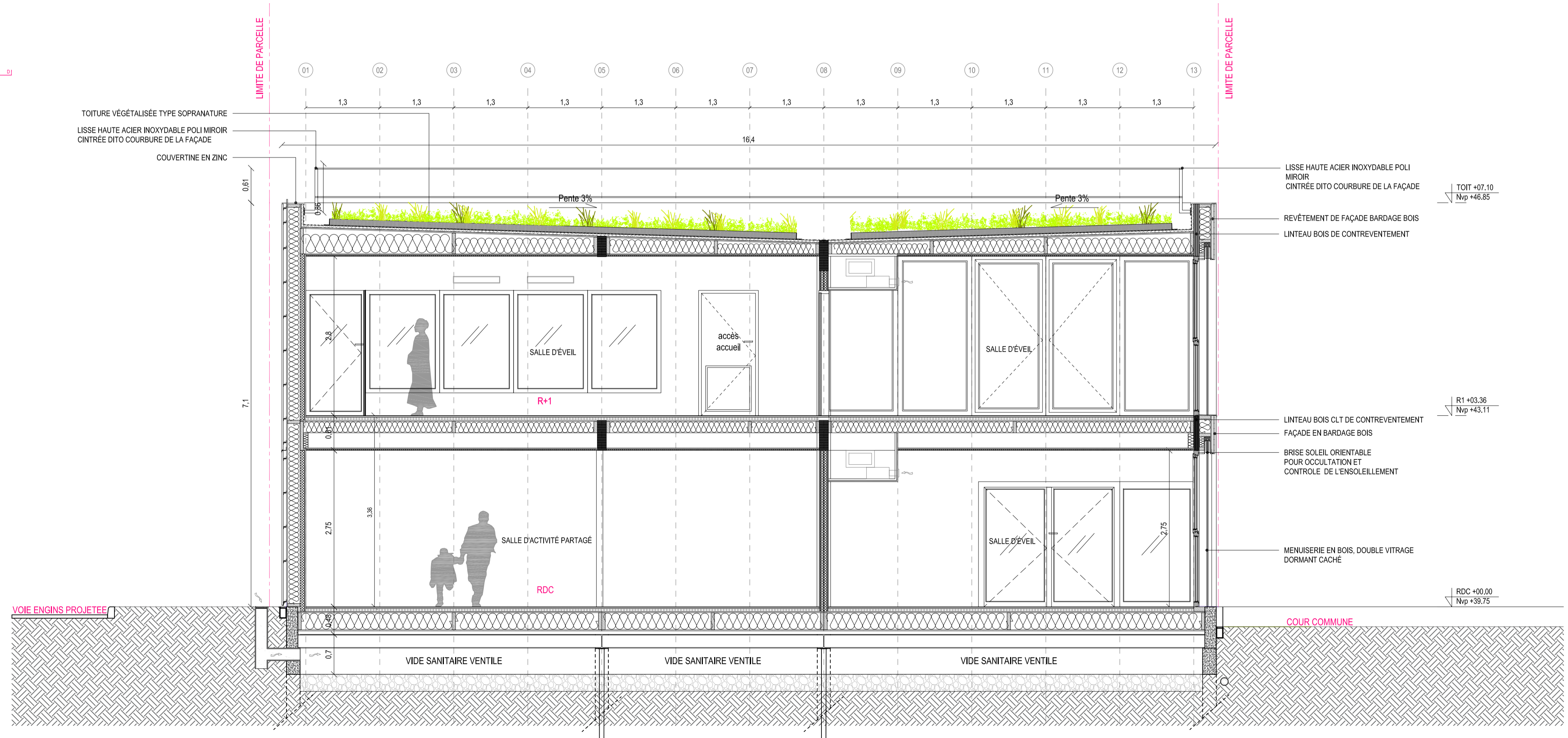
COUPE TRANSVERSALE DD
