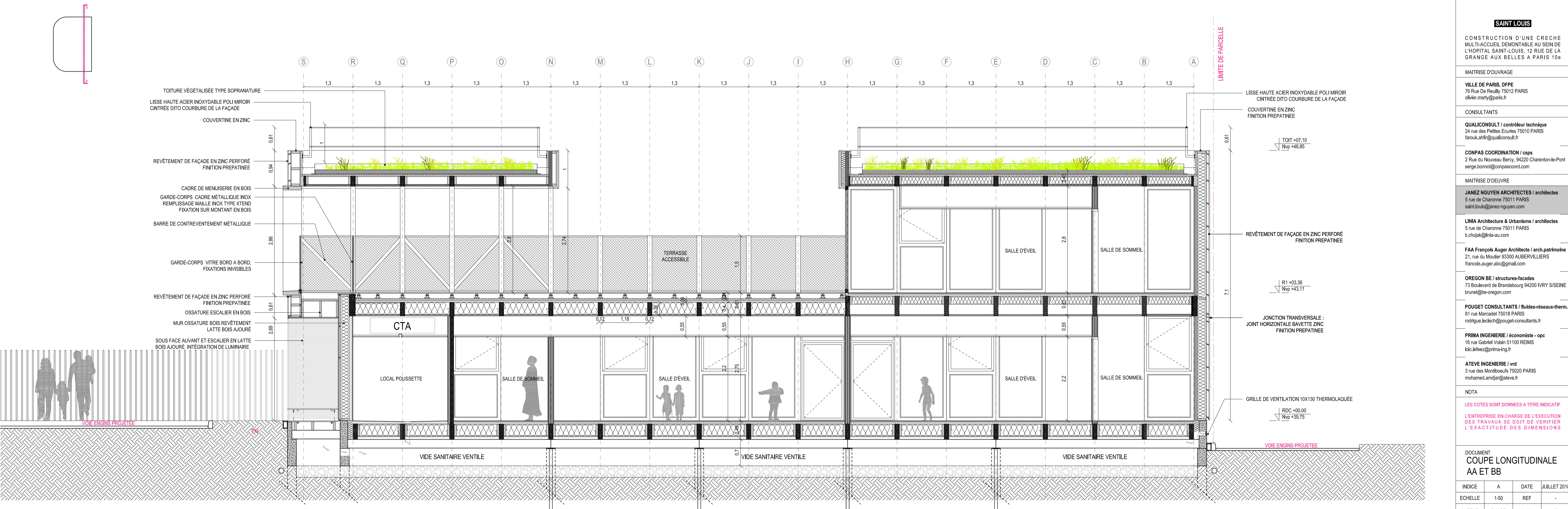
COUPE LONGITUDINALE BB
