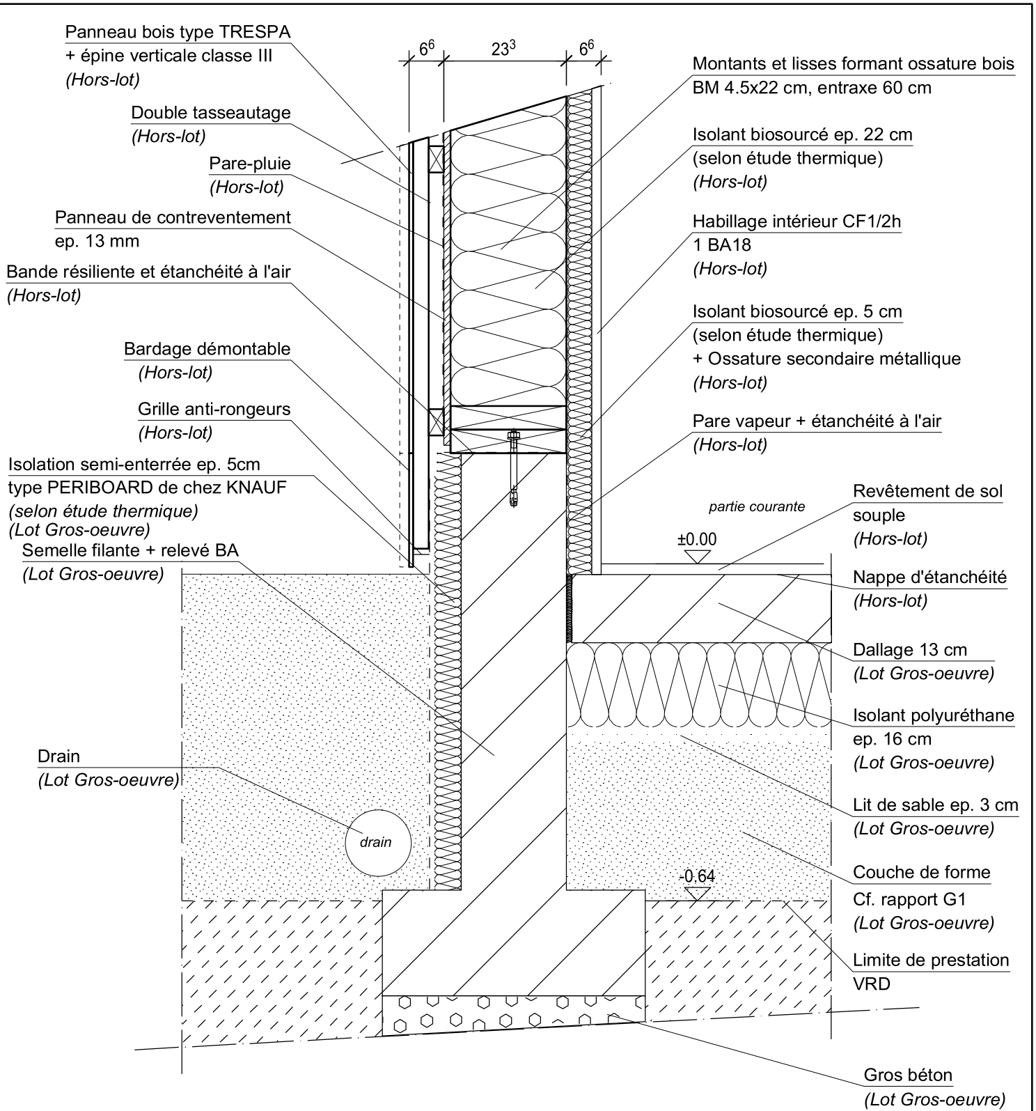
Coupe verticale
