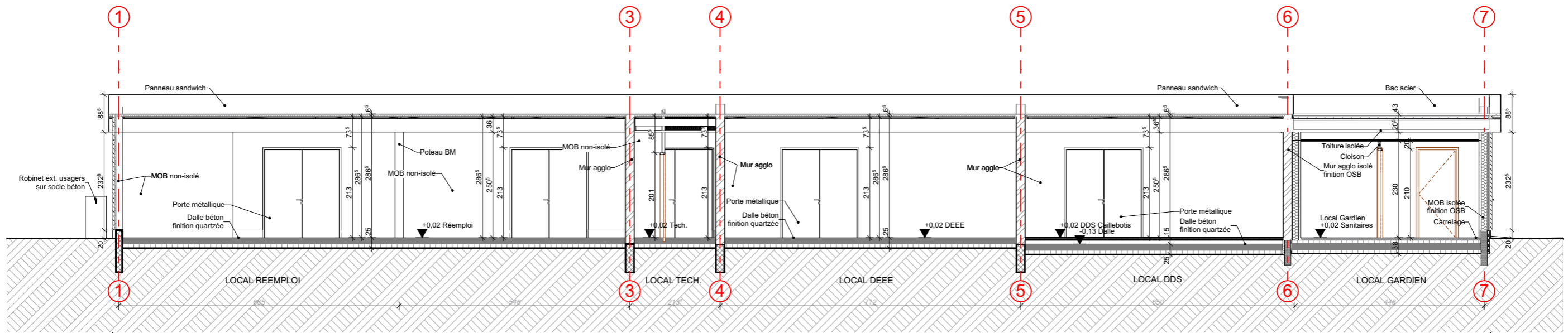
Coupe AA
