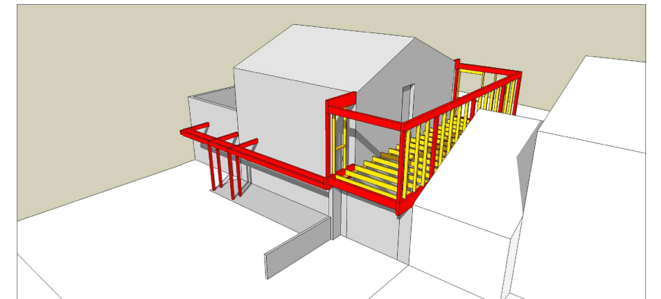
Ossature bois
