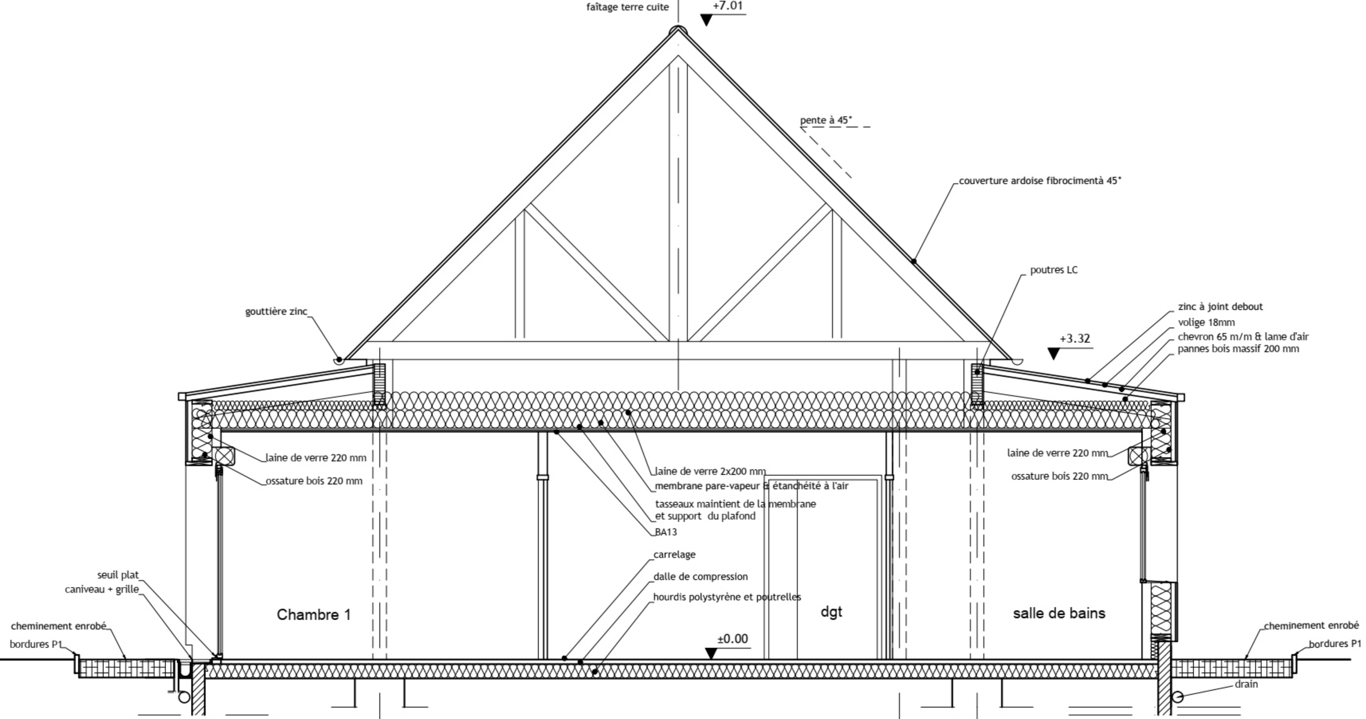
Coupe I-I
