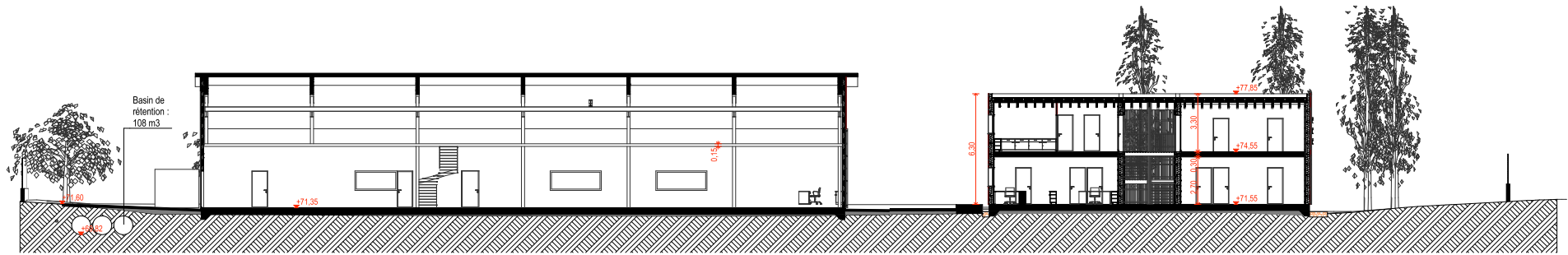
Coupe Longitudinale
