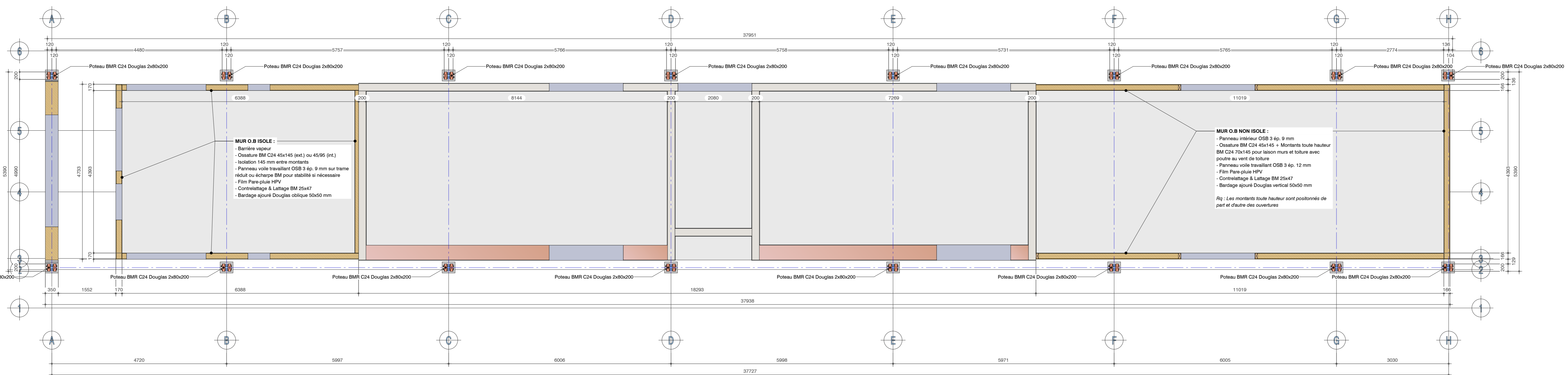
VUE EN PLAN NIVEAU +1.0m - Ech 1/50°
