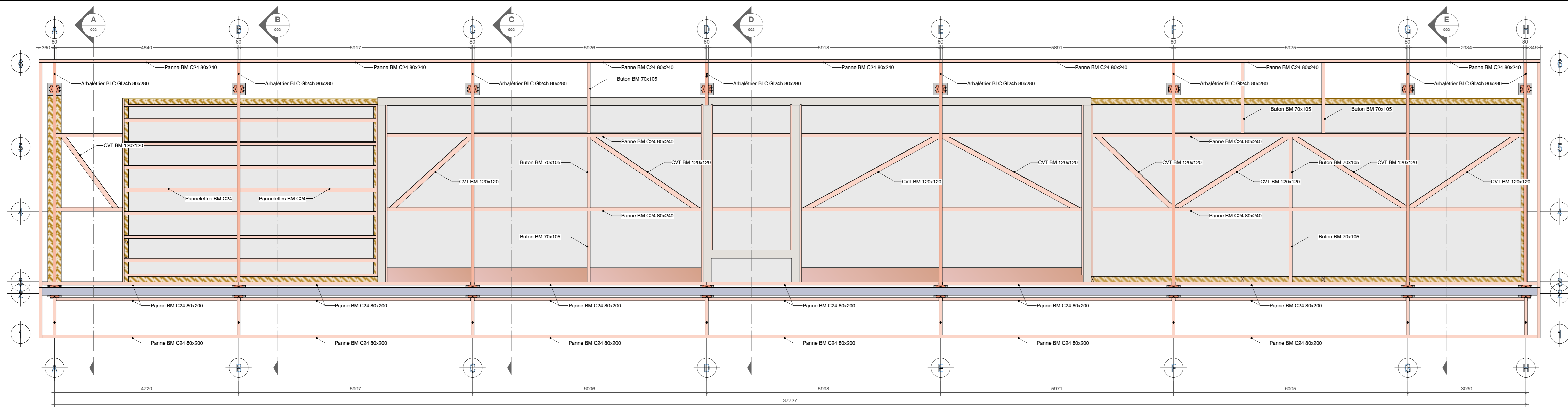
VUE EN PLAN CHARPENTE - Ech 1/50°
