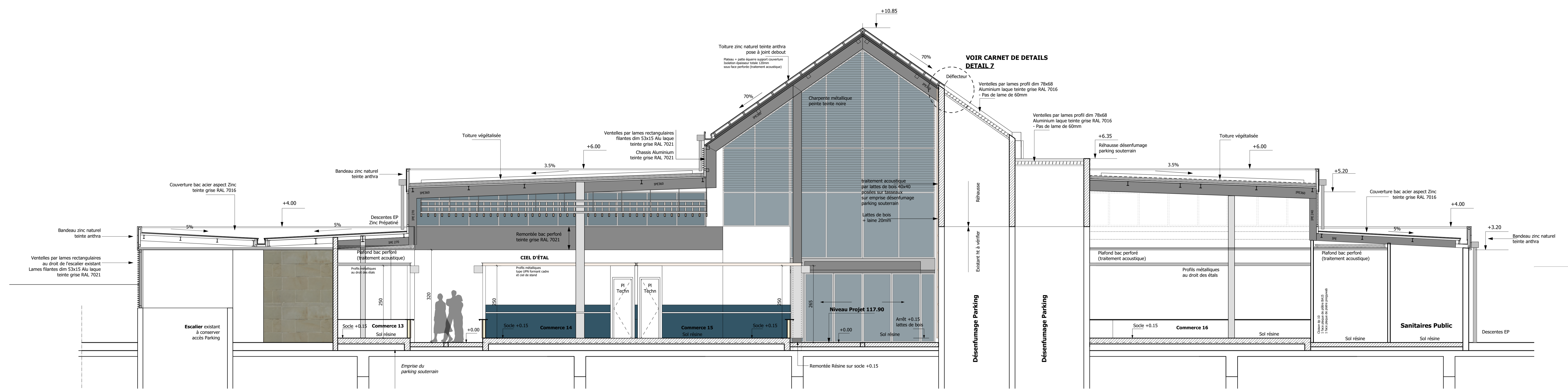
Coupe BB
