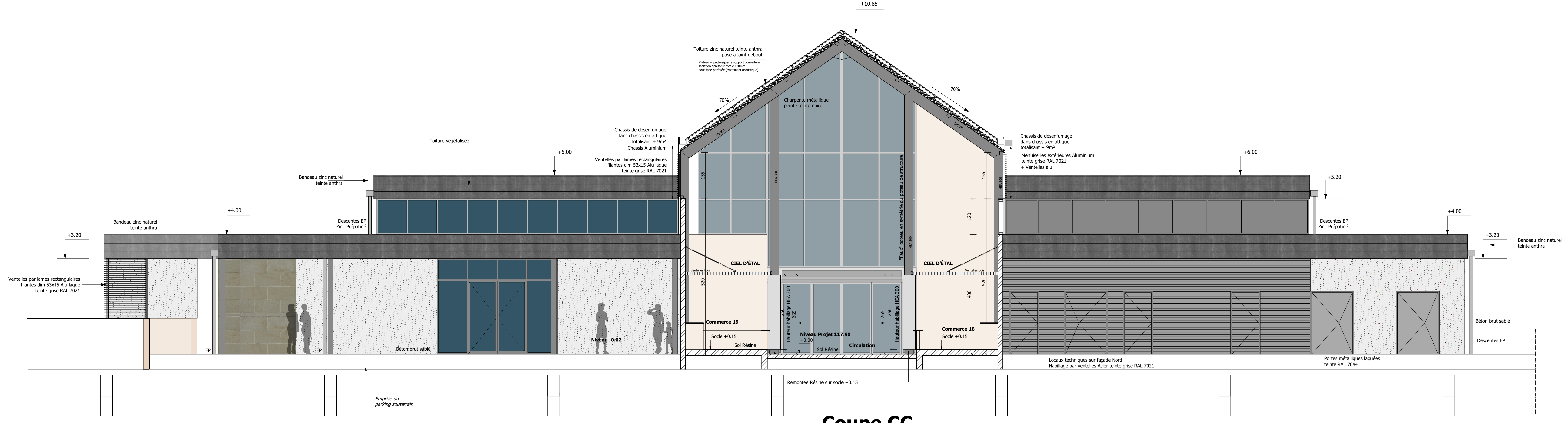
Coupe CC
