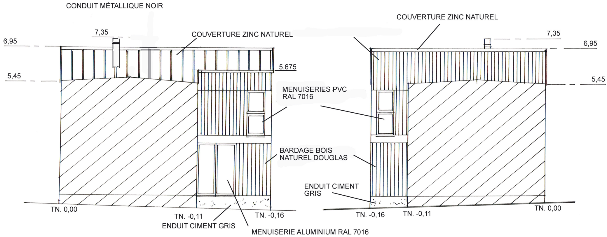
COUPE FACADE OUEST - ECH. 1/100
