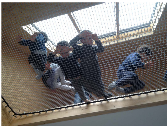
Filet de catamaran sur la mezzanine de l'extension
