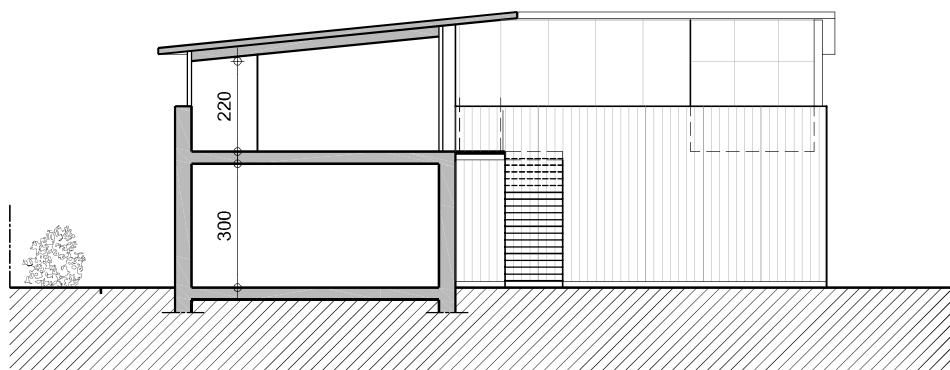
Coupe CC
