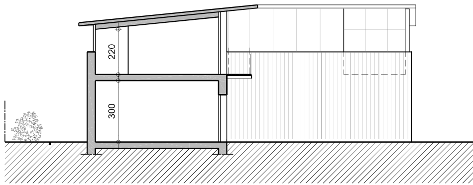
Coupe BB
