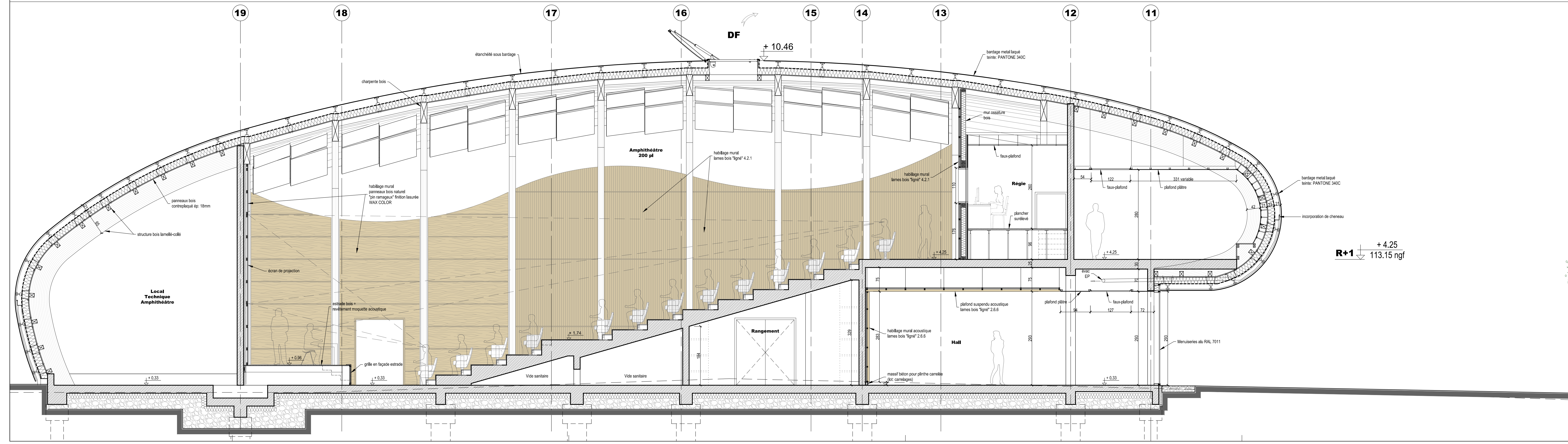
COUPE I ech: 1/50°
