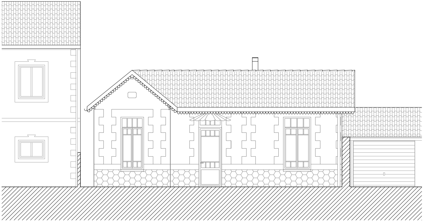
Elévation Sud-Est existant
