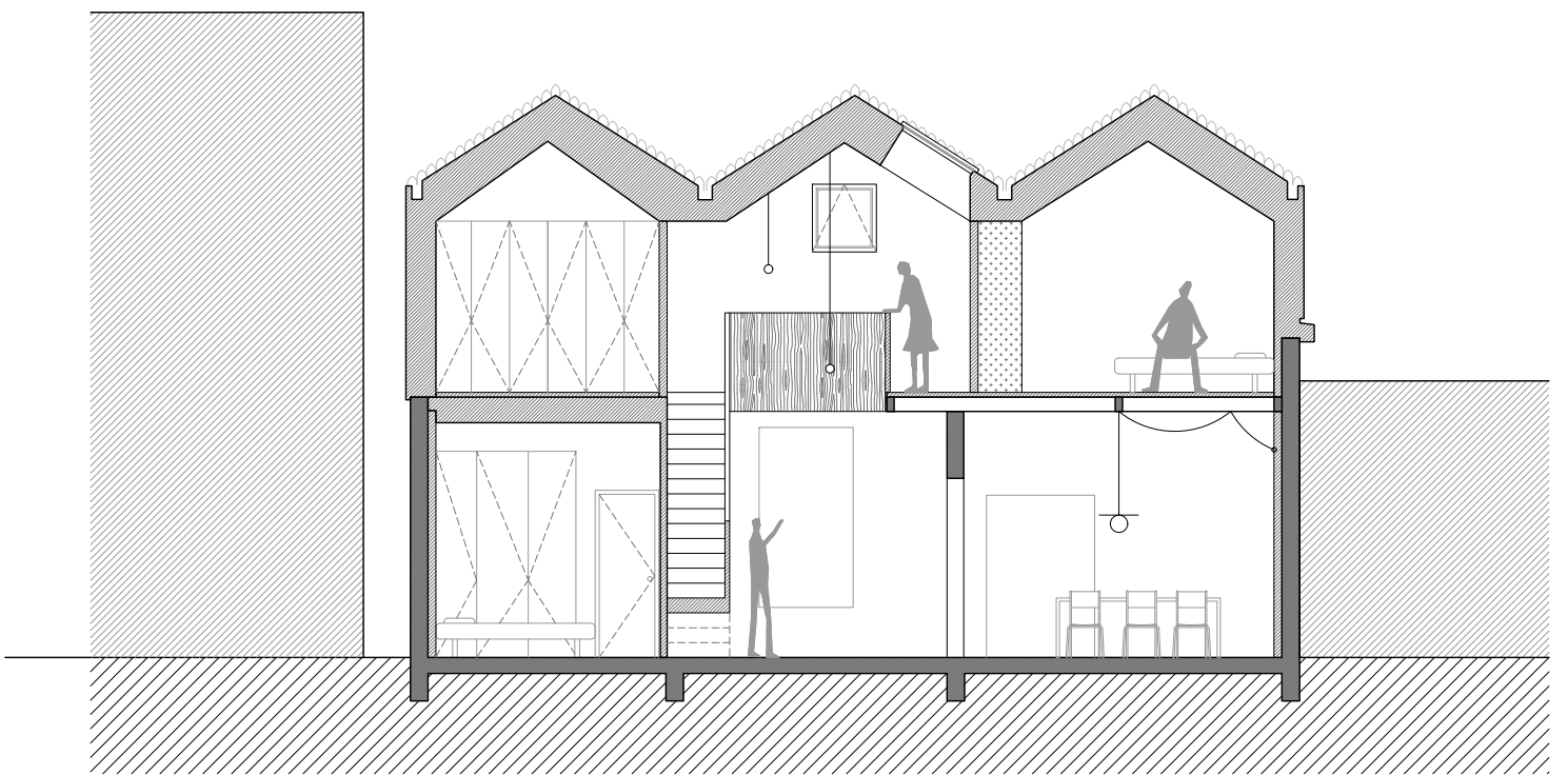
Coupe projet
