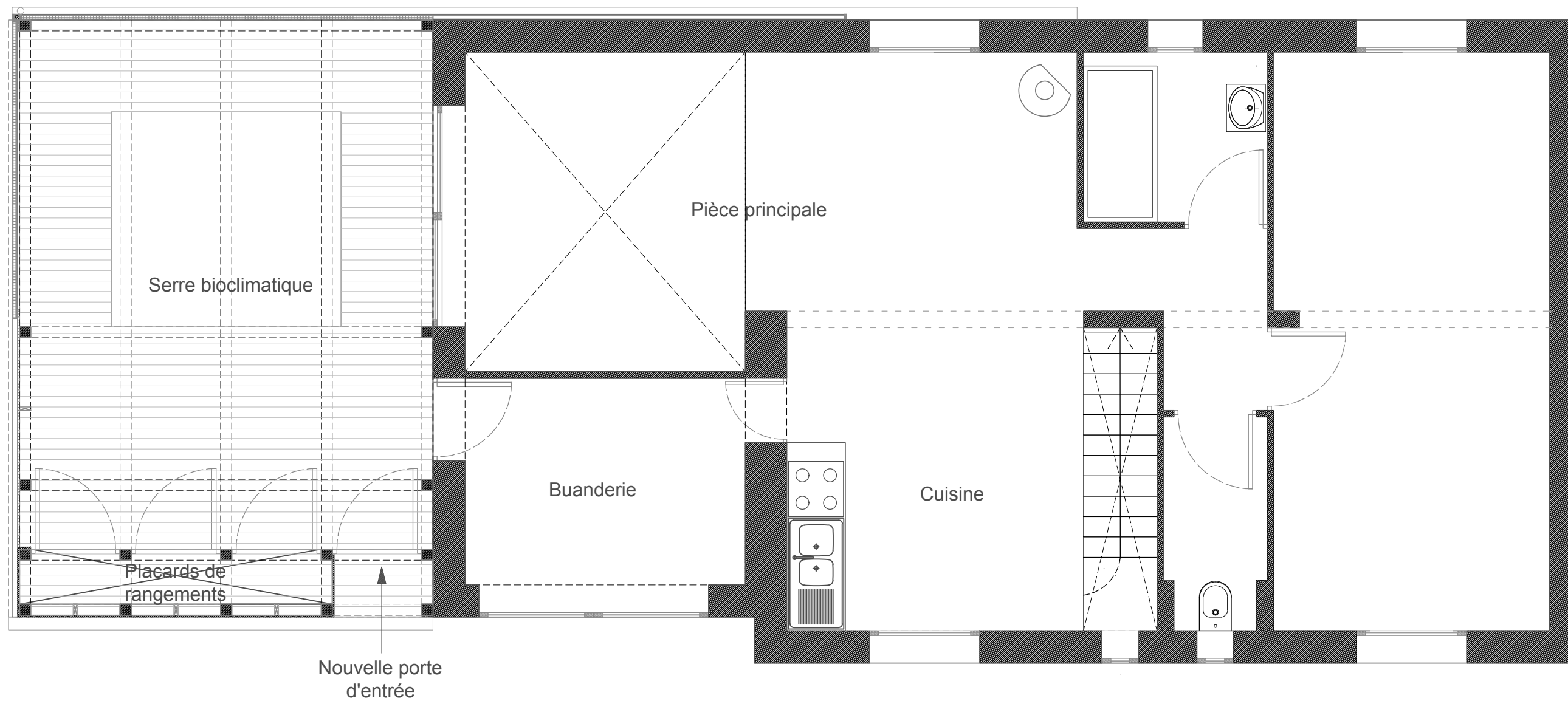
Plan du rez-de-chaussée après la réhabilitation
