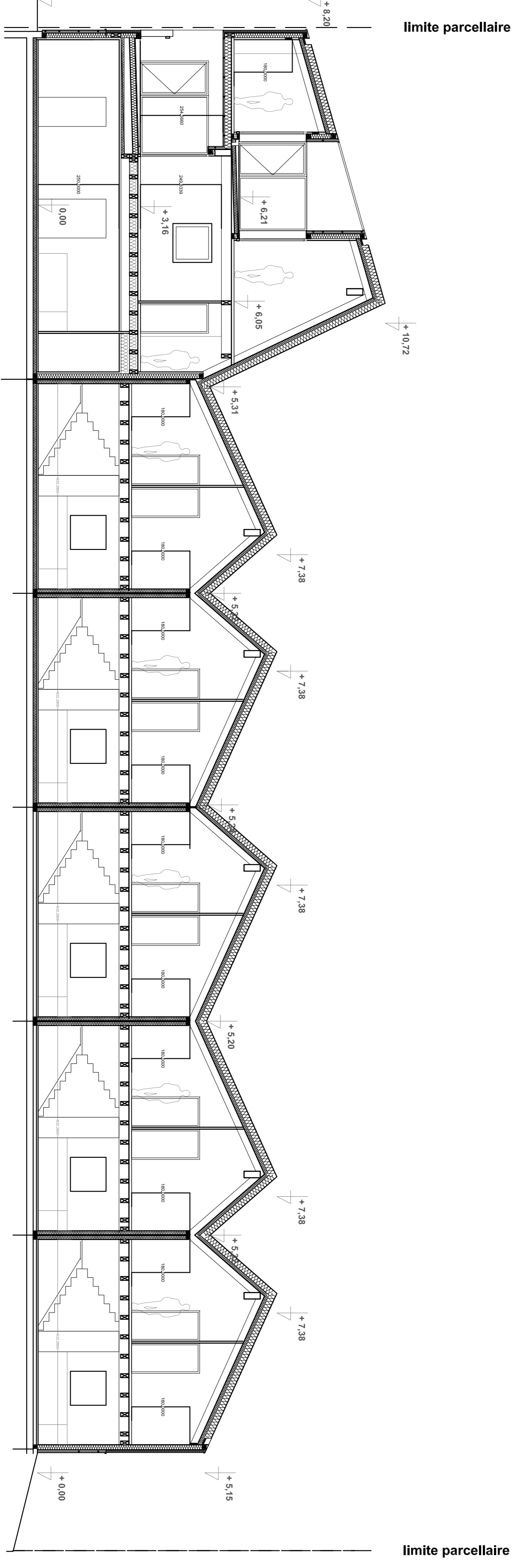
coupe AA
