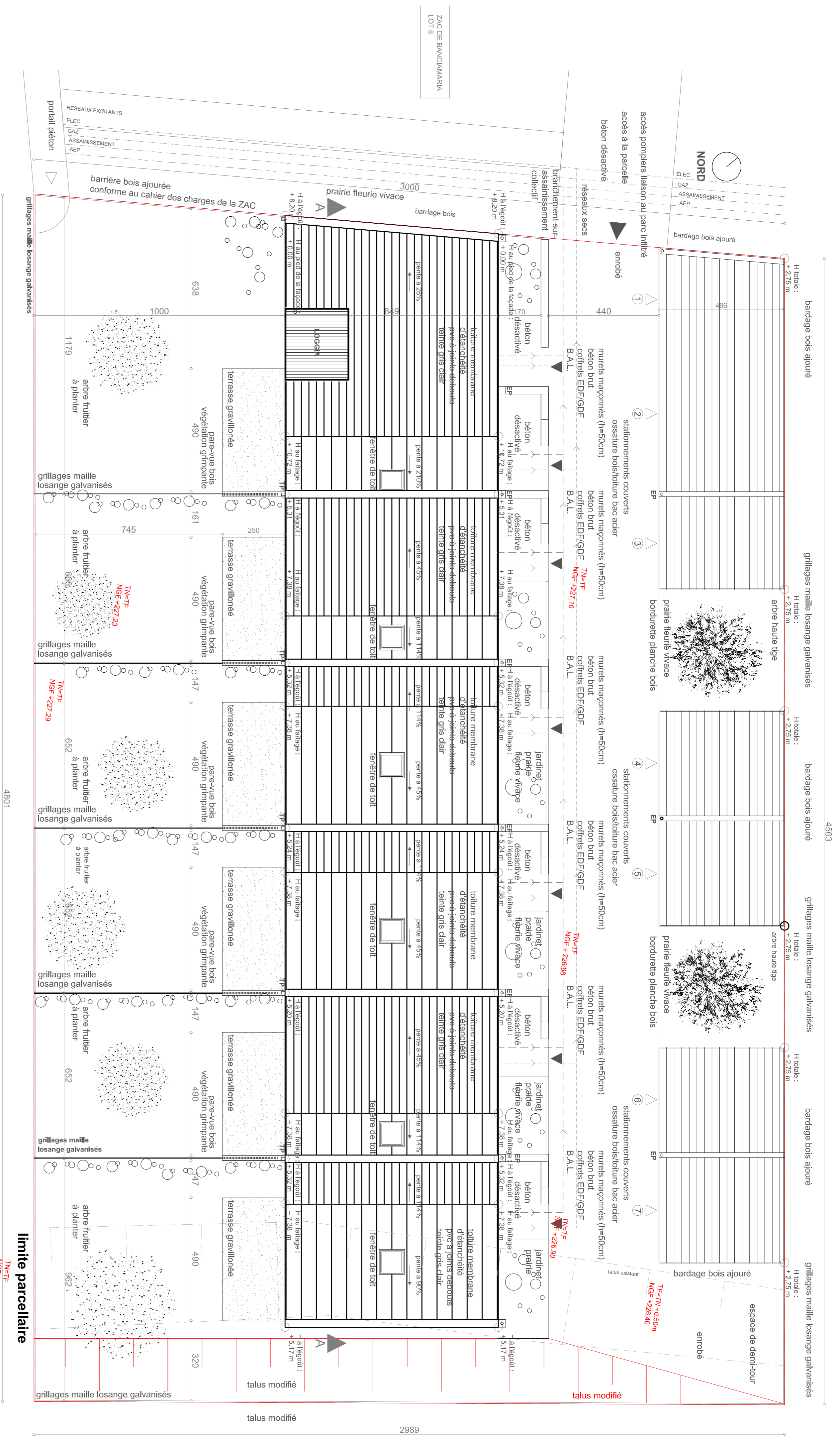
PLAN MASSE _1/100°
