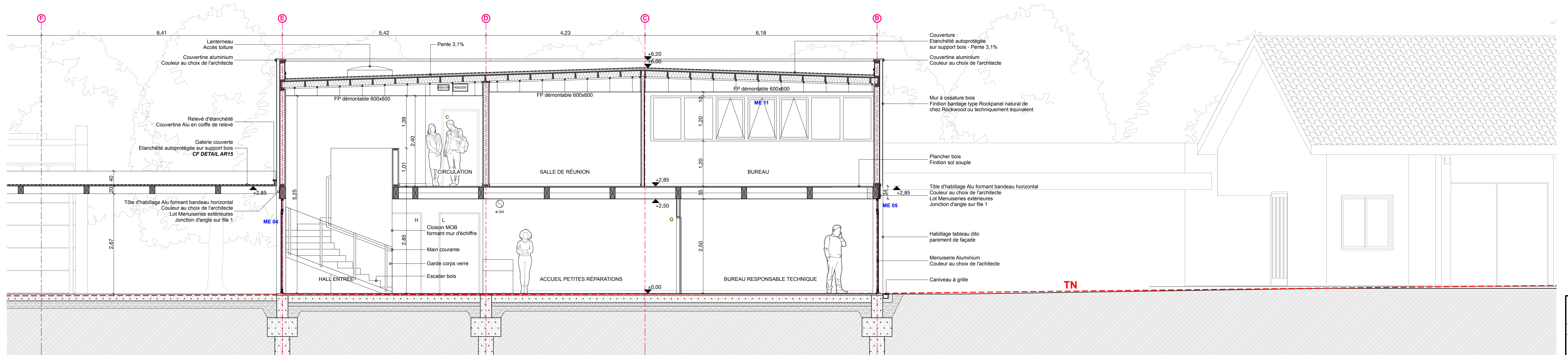
COUPE B
