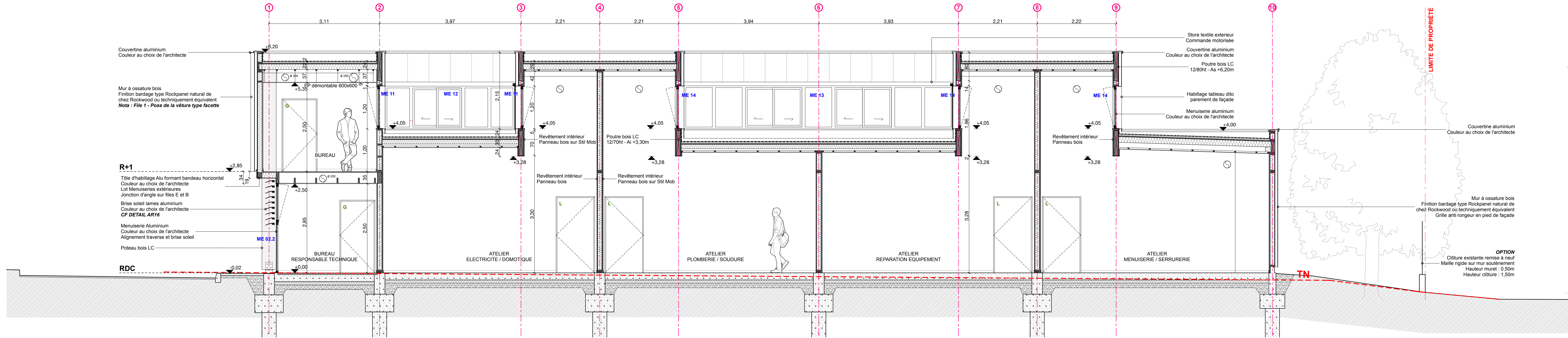
COUPE A
