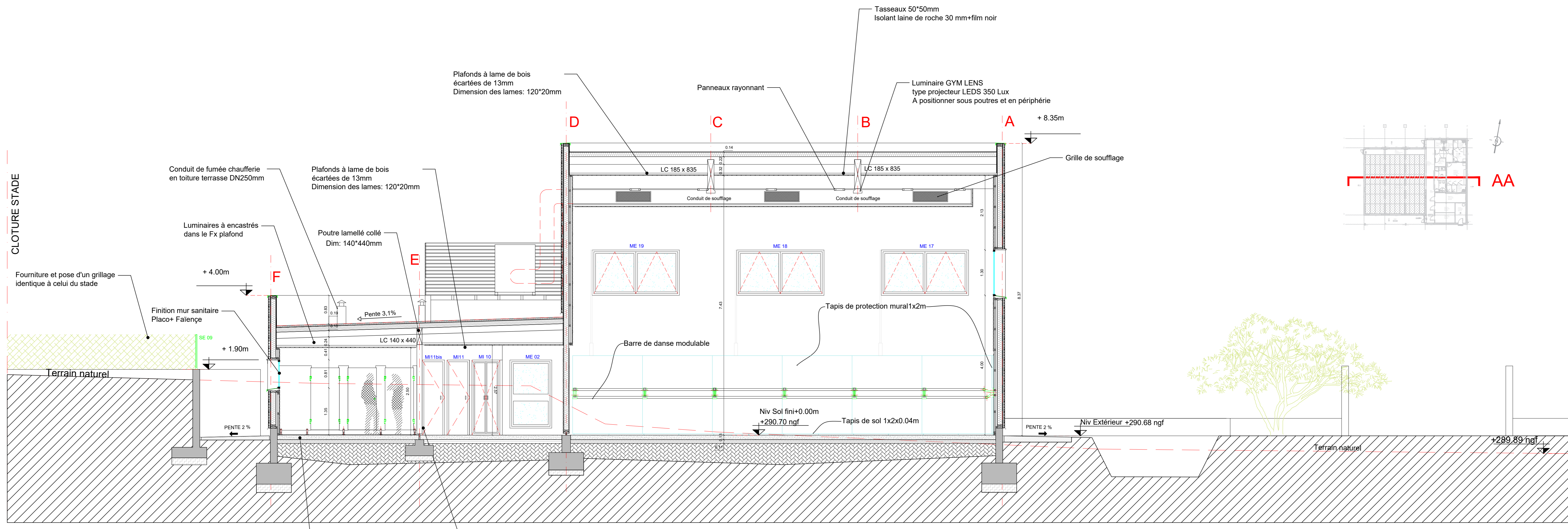
Coupe AA Projet 0.00 = 290.70 NGF
