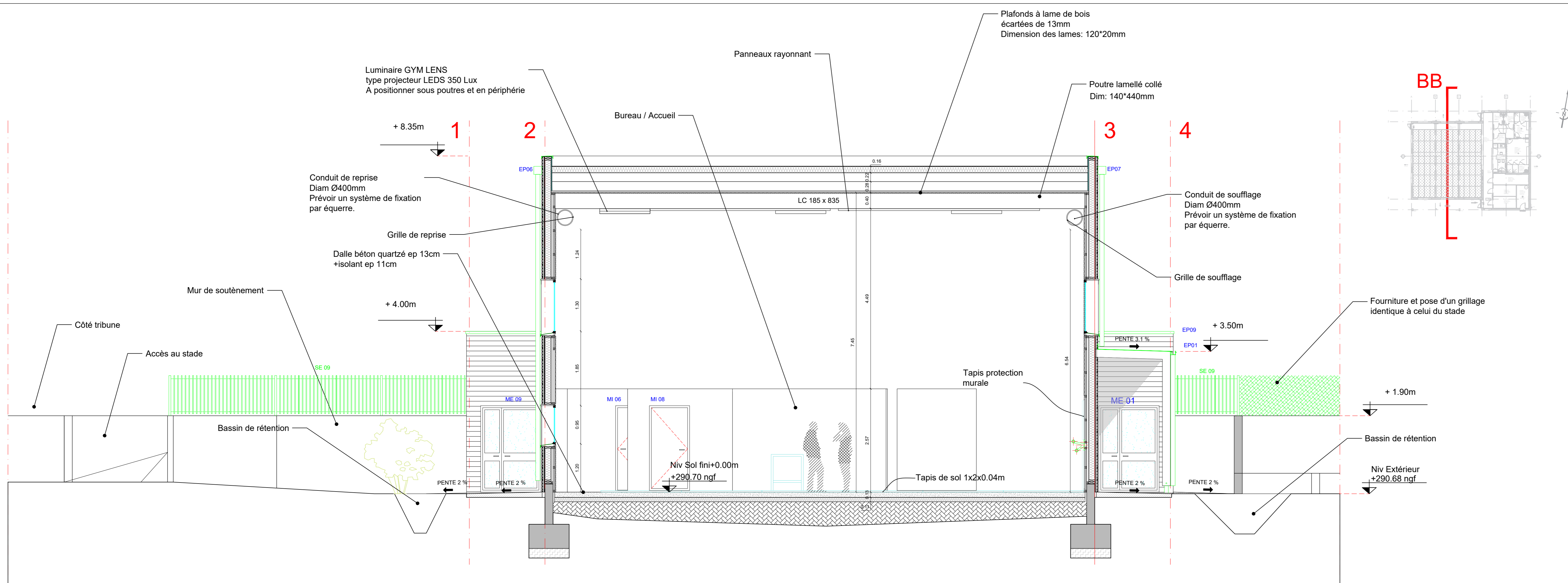
Coupe BB Projet 0.00 = 290.70 NGF
