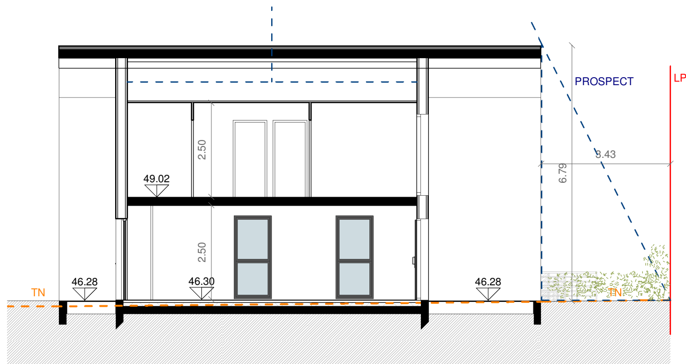
Coupe B-B' (M8)
