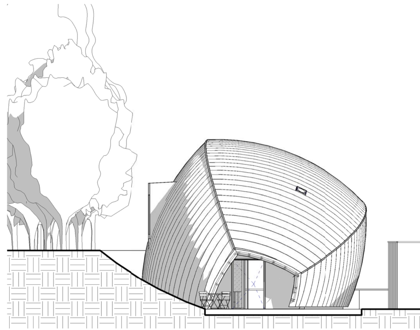
Élévation Nord-Est_BIENNALE Ech : 1 : 100
