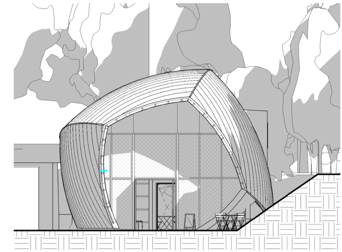
Élévation Sud-Ouest_BIENNALE Ech : 1 : 100
