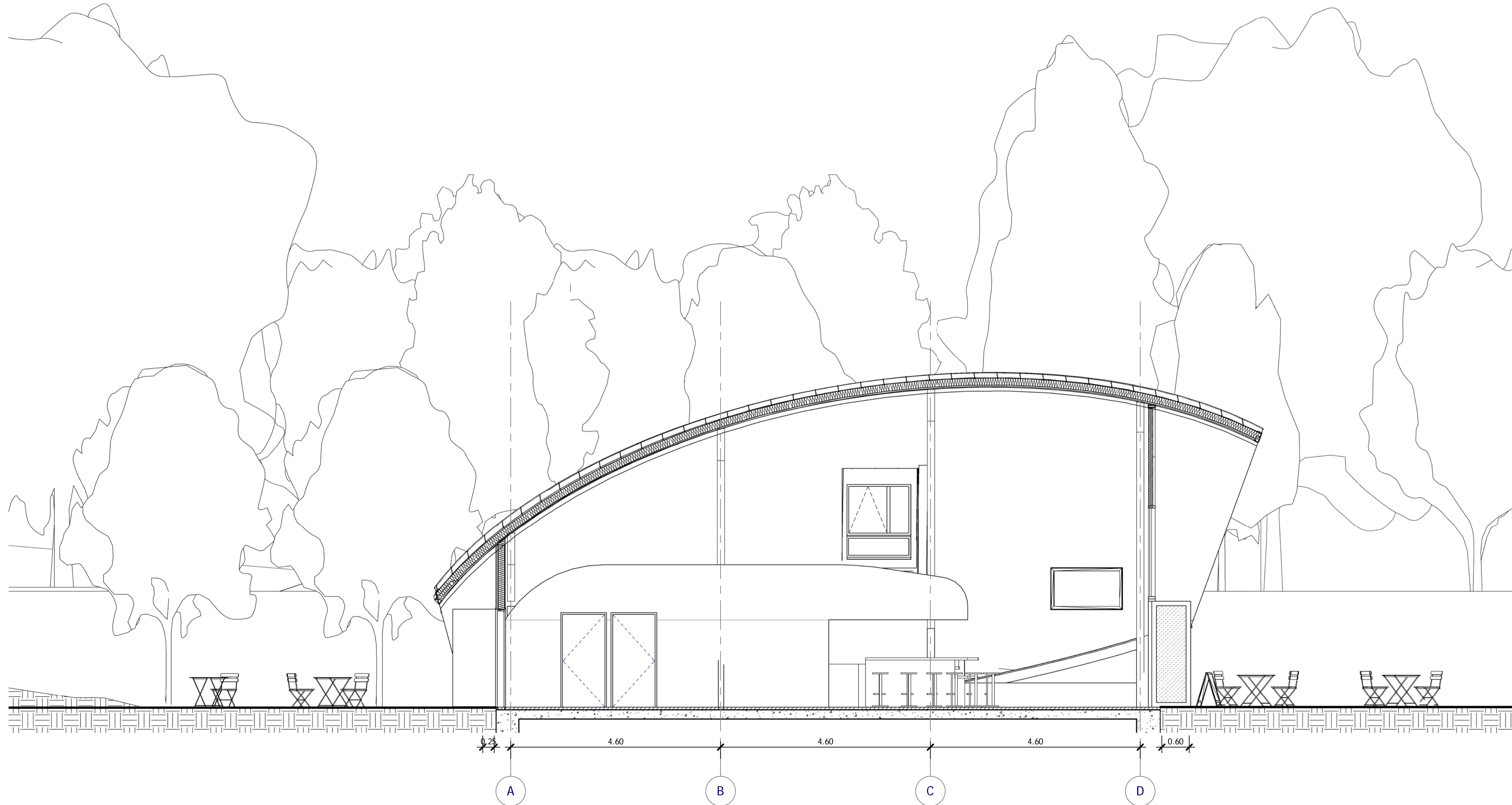
PLA_Coupe A-A_BIENNALE Ech : 1 : 50
