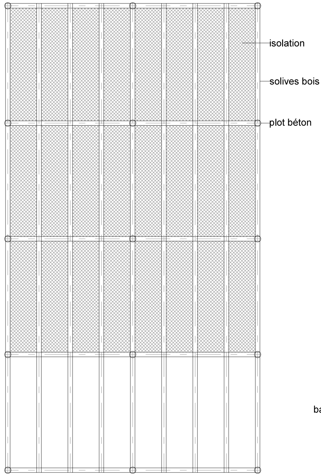
PLAN DE PRINCIPE PLANCHER BOIS
