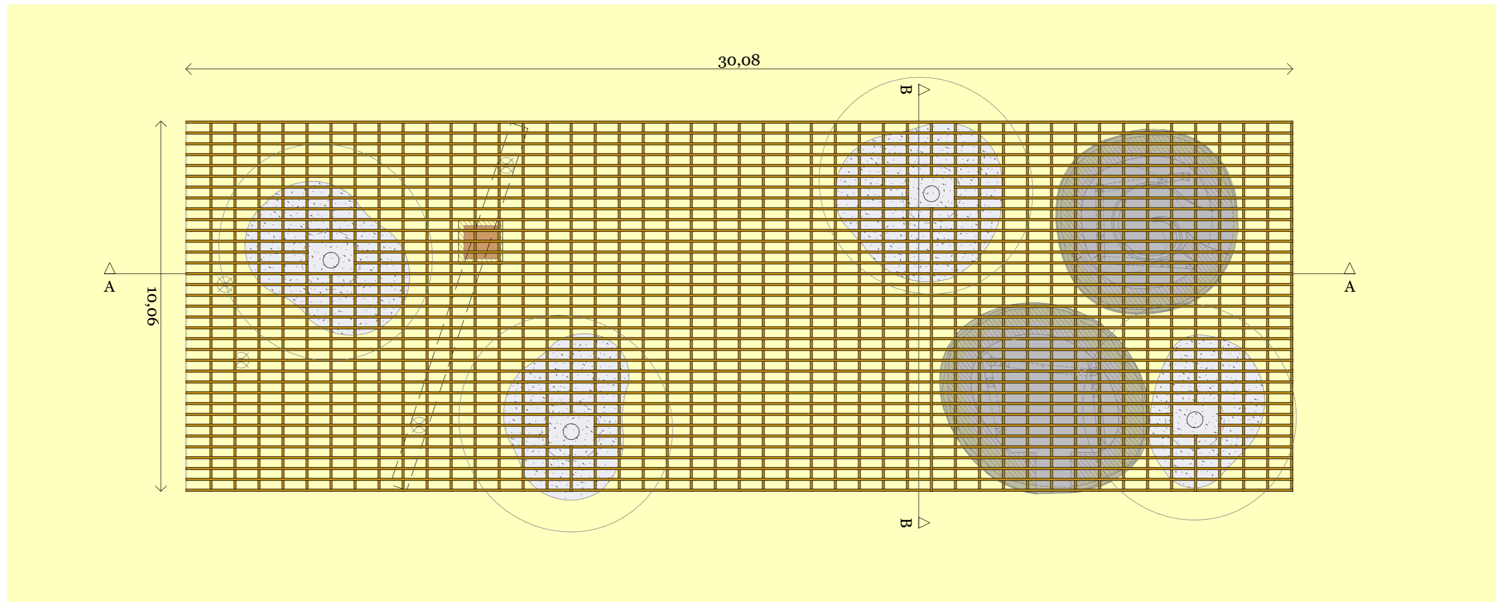
PLAN AU SOL - 1:200
