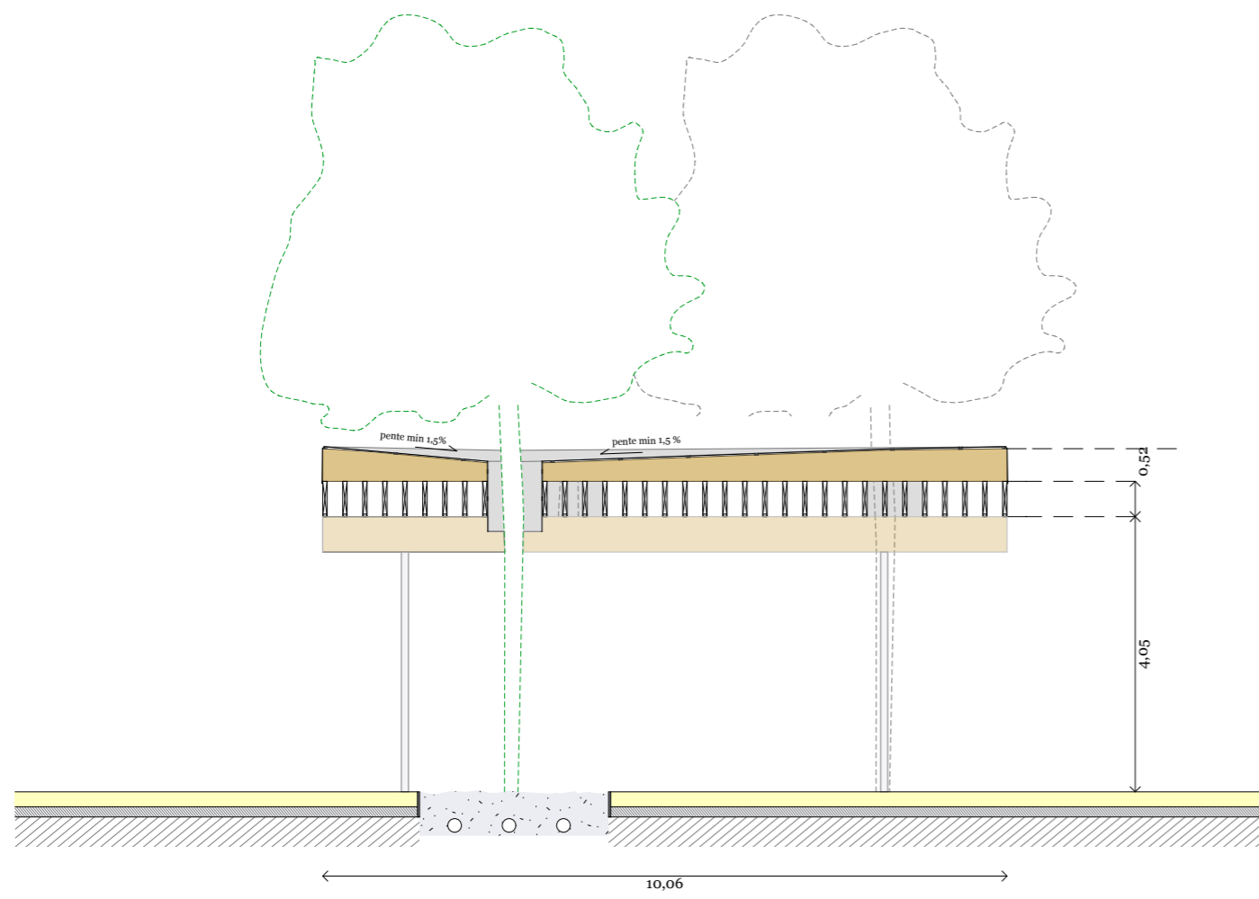
COUPE BB - 1:100
