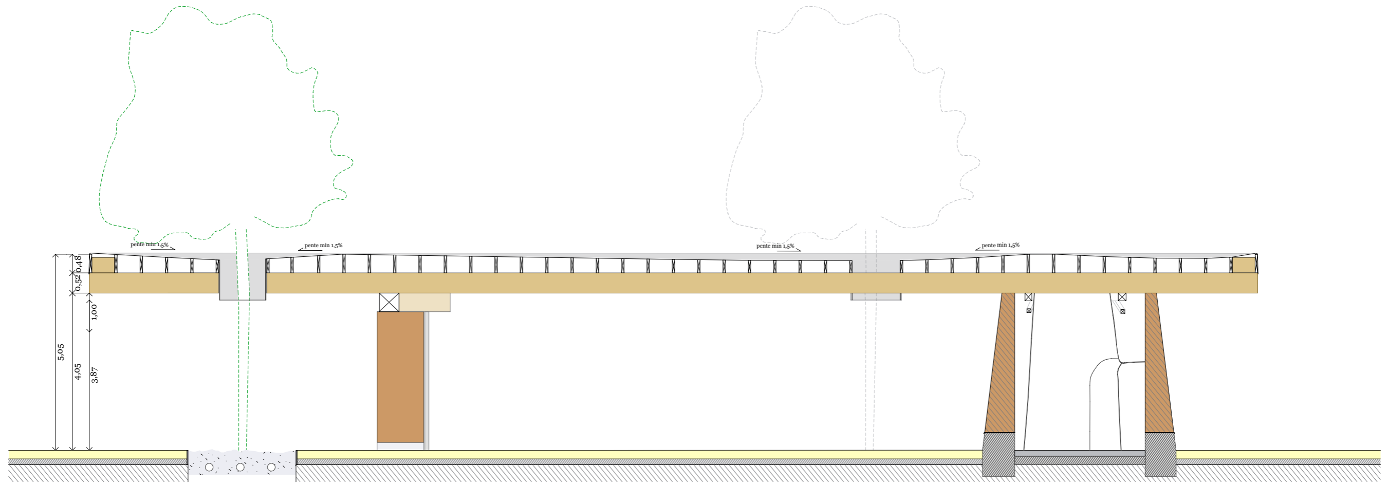
COUPE AA - 1:100
