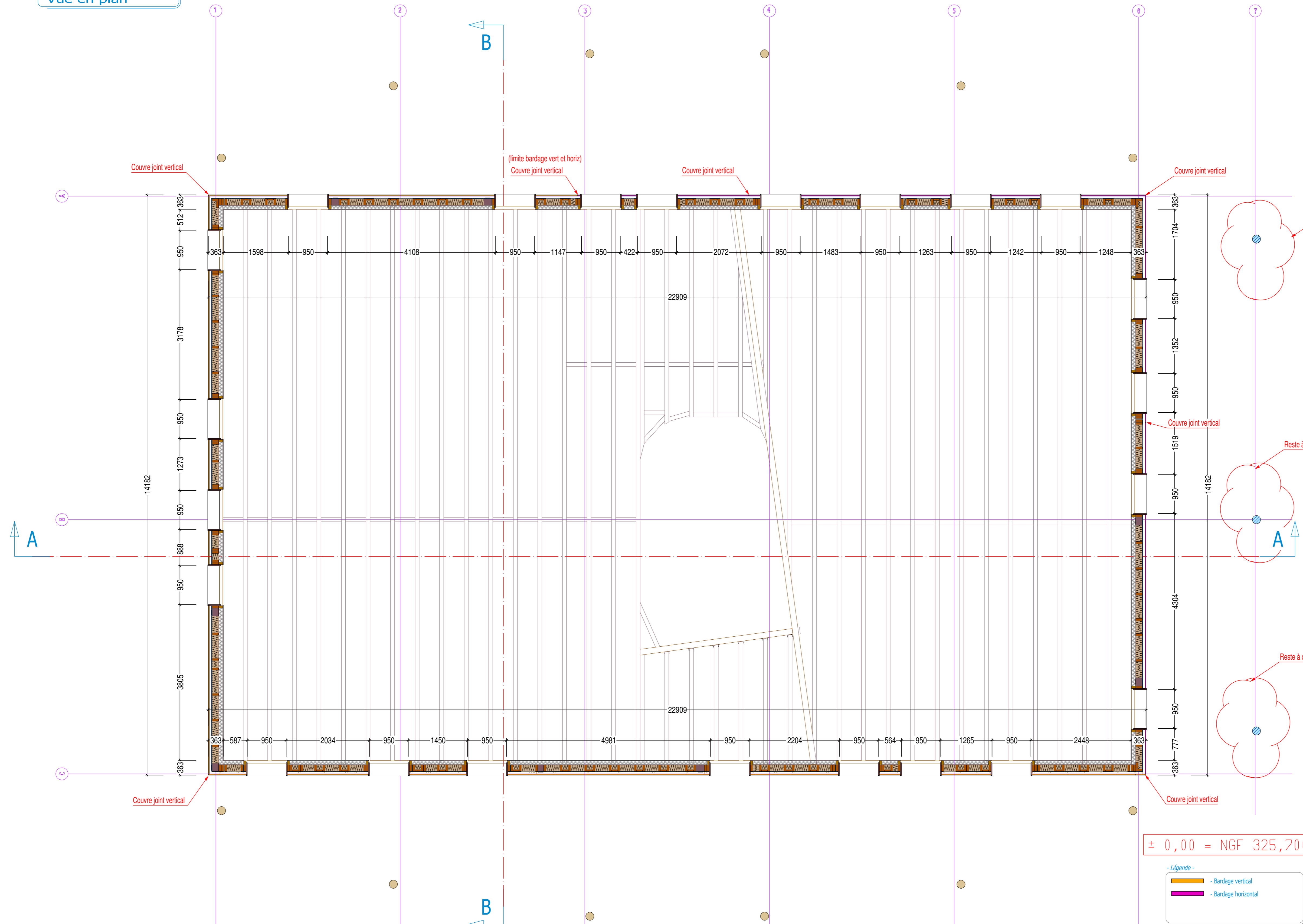
Vue en plan Ech: 1/50
