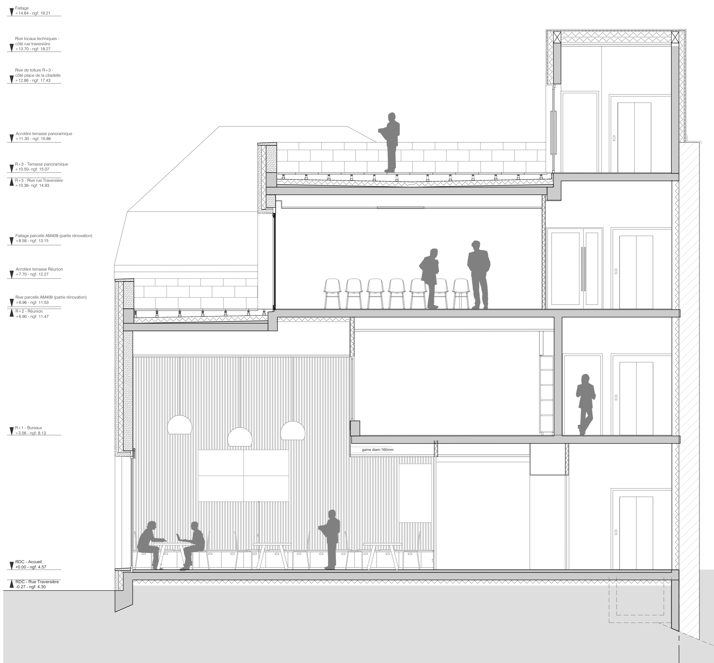
Coupe AA'
