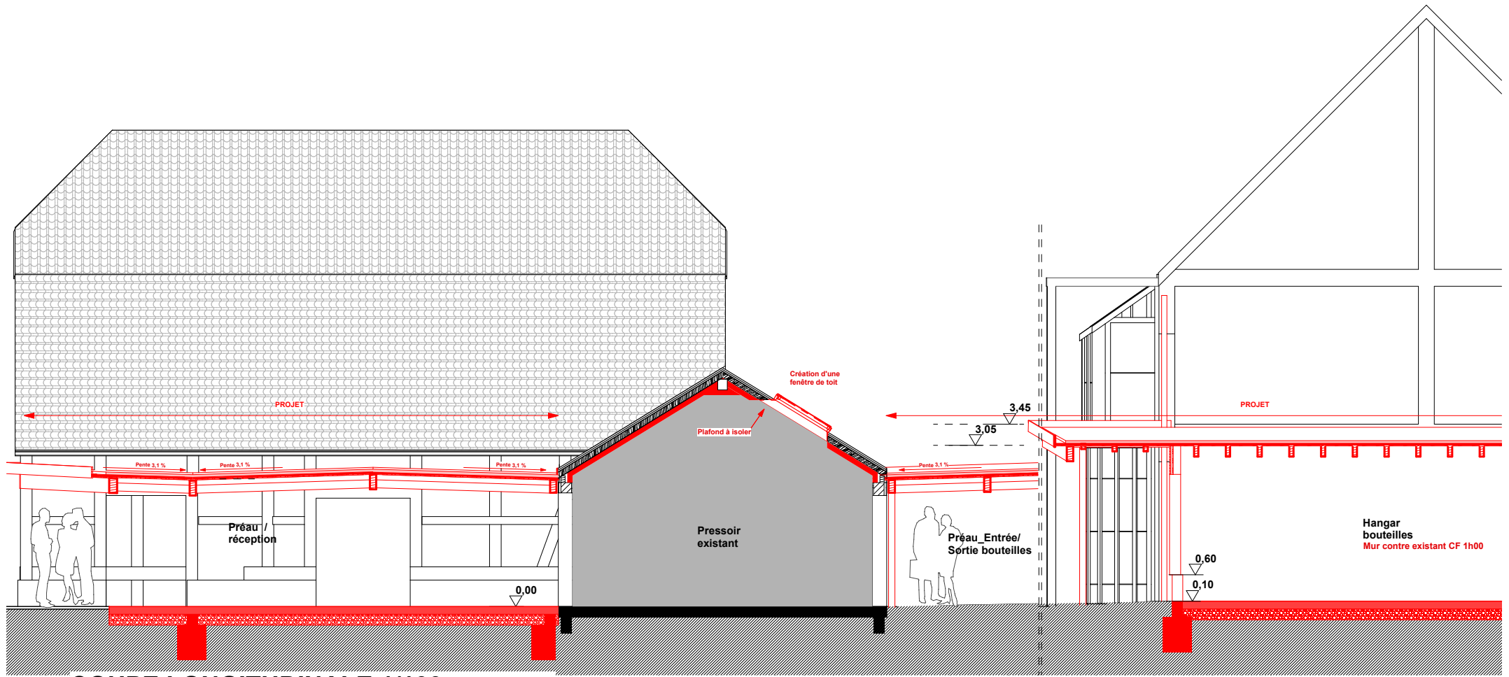
COUPE LONGITUDINALE 1/100
