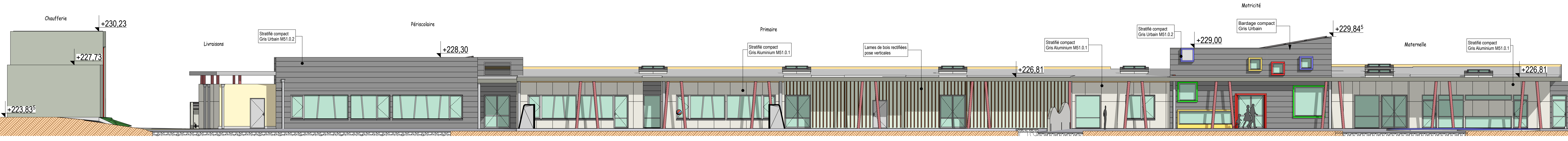
ELEVATION FACADE NORD EST éch 1/100
