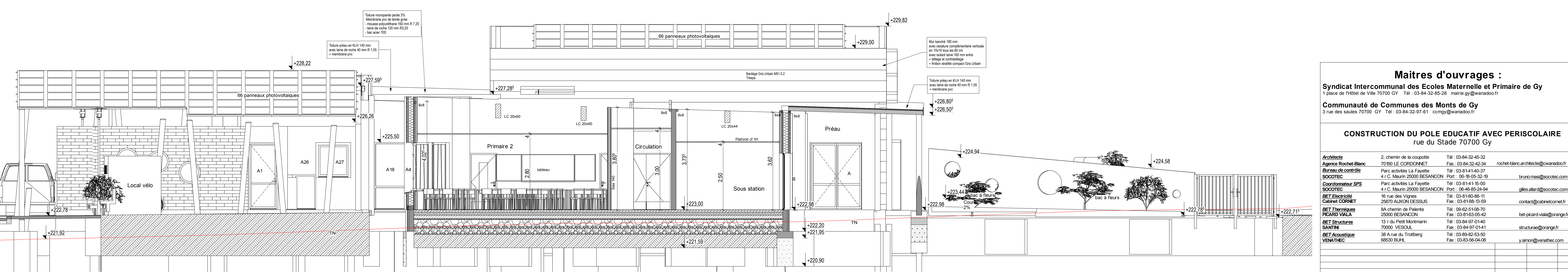
COUPE SUIVANT A3 éch 1/50°
