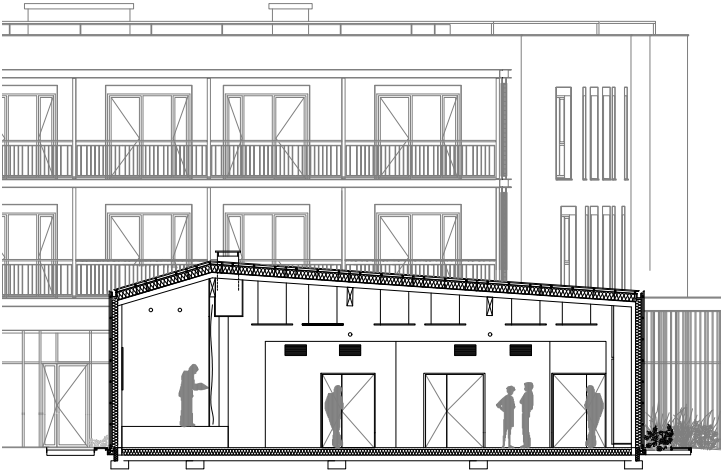
COUPE LONGITUDINALE
